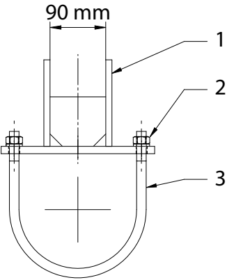
Ablagebock H 1 für Auslegerabspannung
