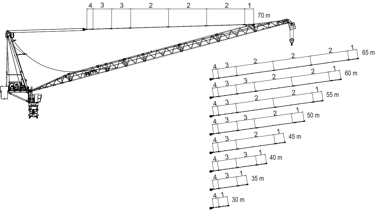
Abspannungsaufstellung
