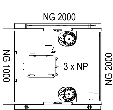
Normgeländeranordnung Drehrahmen
