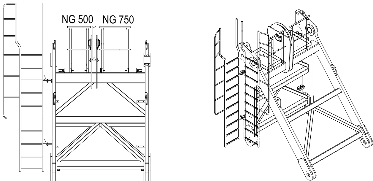
Normgeländeranordnung Verbindungsbock
