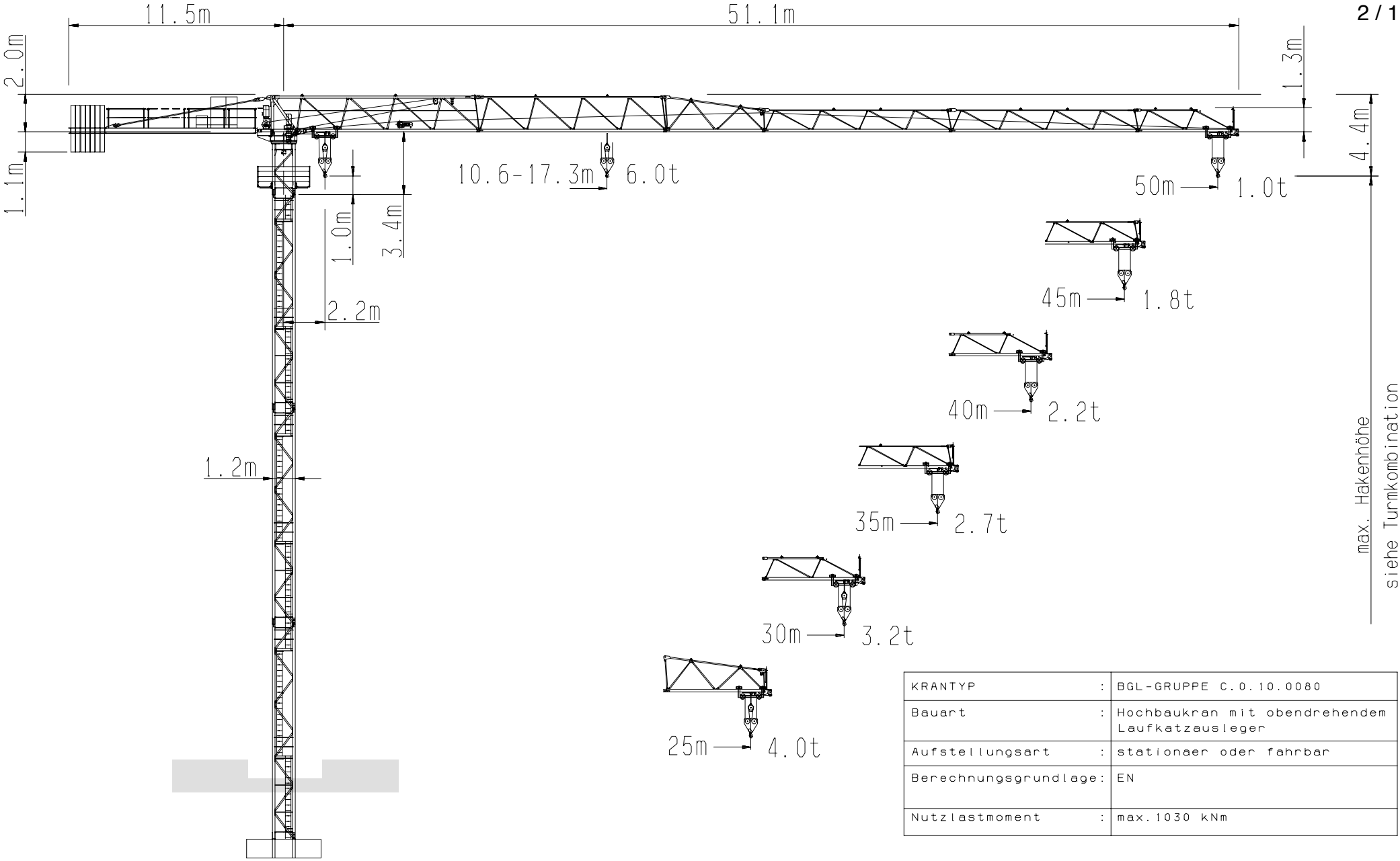
Planungszeichnung WOLFF 4517 city 962-3-028181
