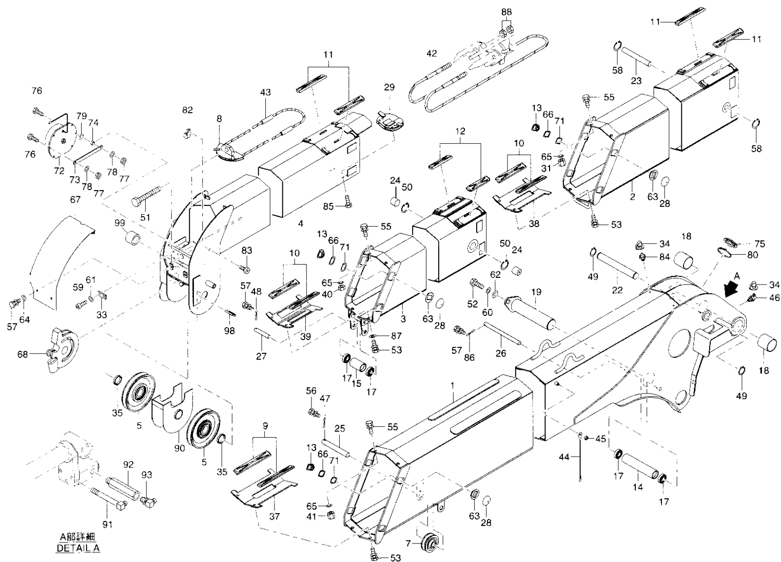
Fig. 1-9 4段ブーム組立(URV374 F仕様) 4-section BOOM ASS'Y(URV374 F type)
