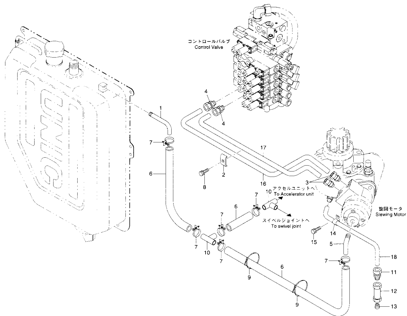
パイピング(旋回モータ)(URV370系 RK 仕様) Fig. 6-3-4 PIPING(Slewing motor)(URV370 series RK type)
