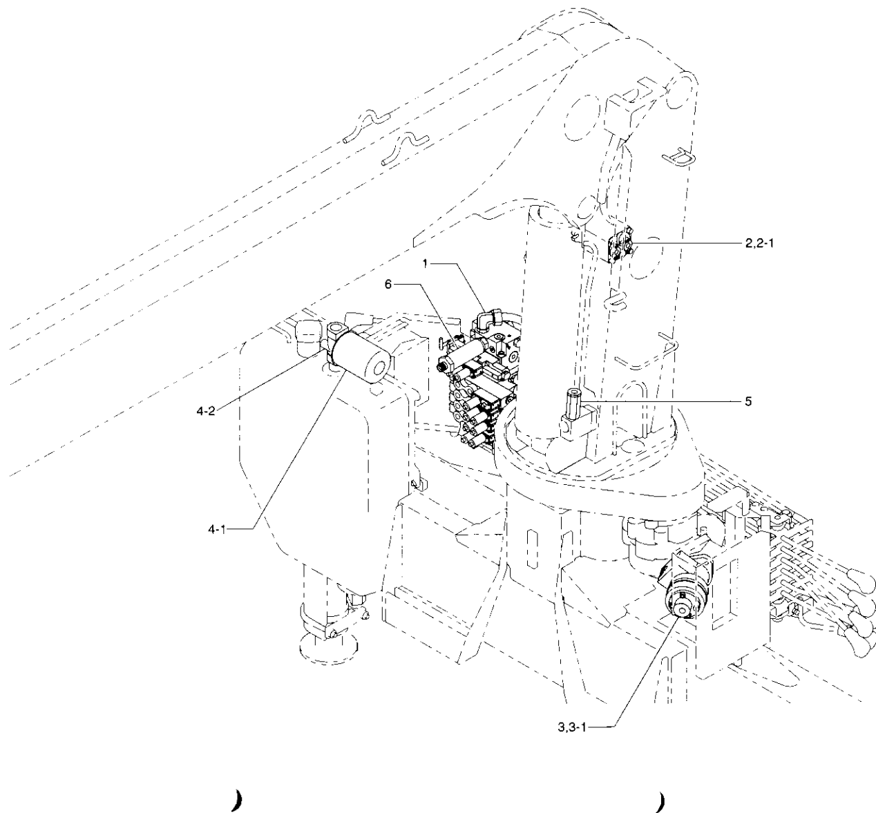
油圧駆動装置(URV370系 R 仕様) Fig. 5-4 HYDRAULIC DRIVING DEVICE(URV370 series R type)
