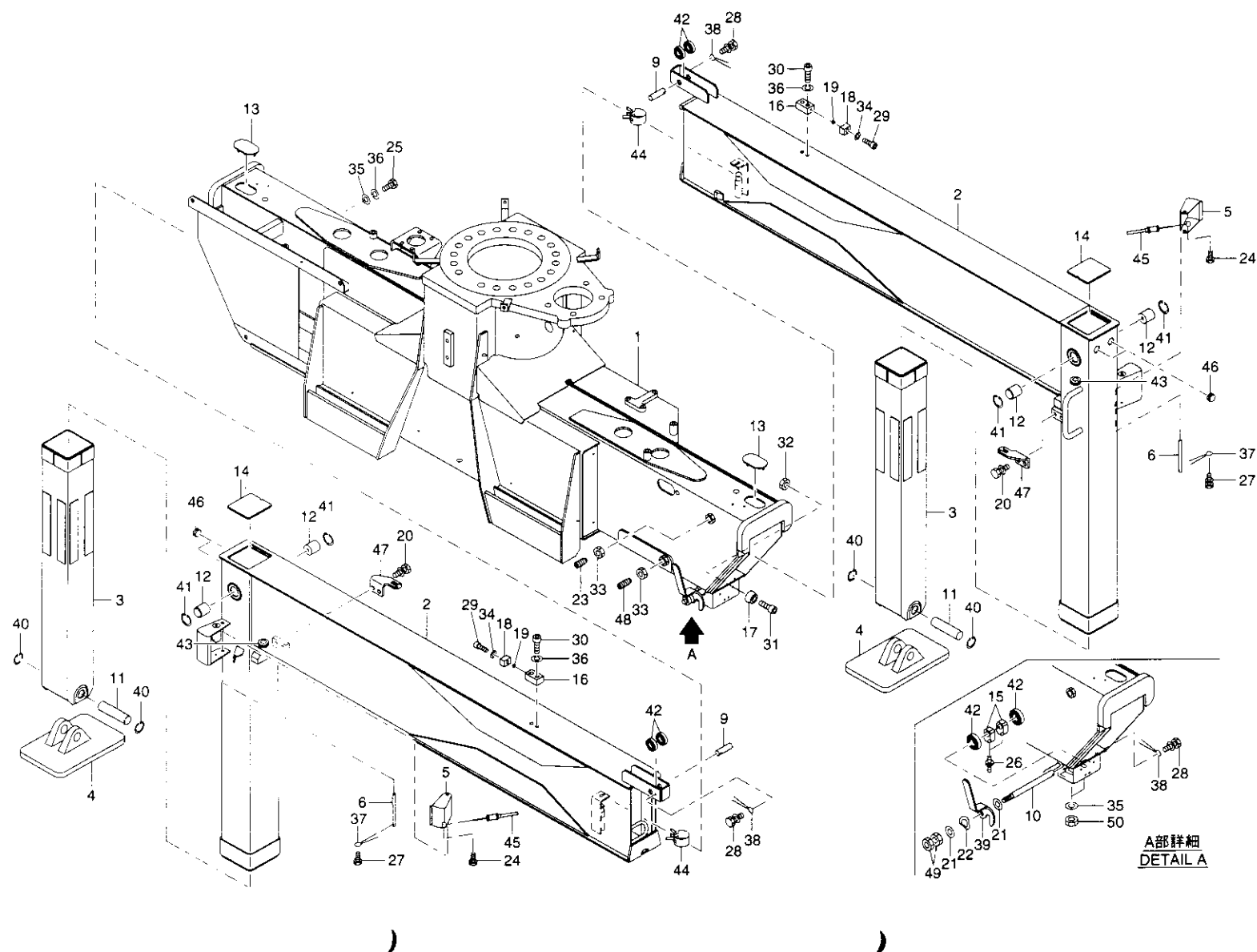
ベース組立(URV370系 GK, G 仕様) Fig. 8-2 BASE ASS'Y(URV370 series GK & G type)
