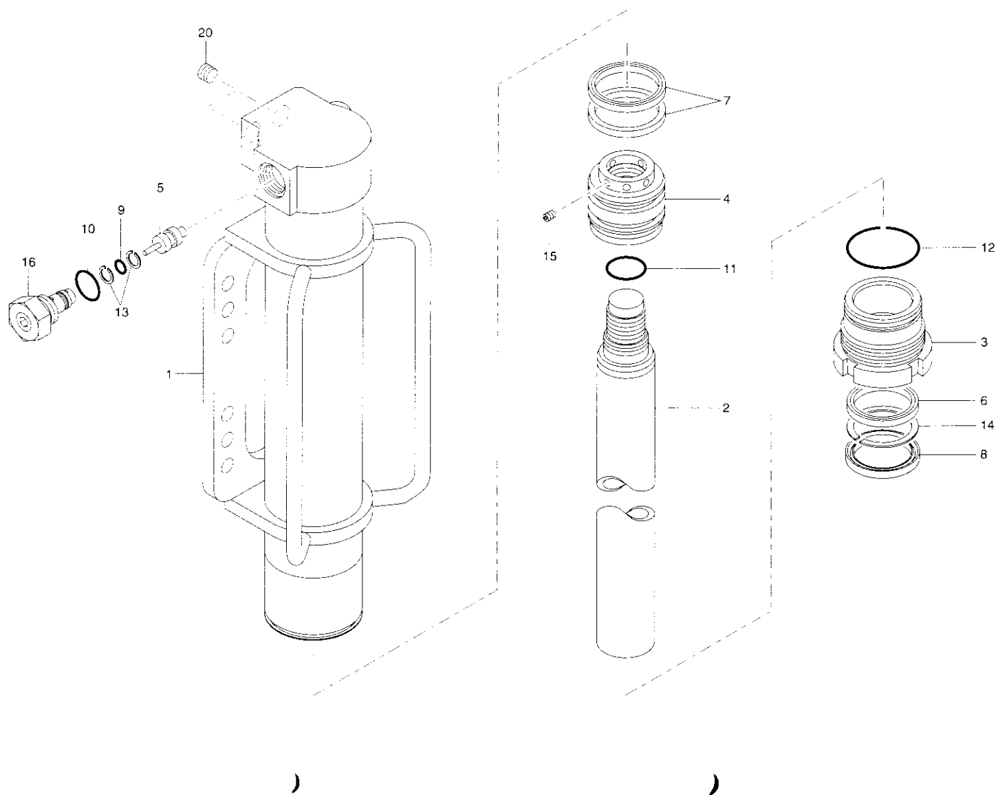
Fig. 20-2 アウトリガシリンダ (リヤ) 組立 (URV376) OUTRIGGER CYLINDER (Rear) ASS'Y (URV376)
