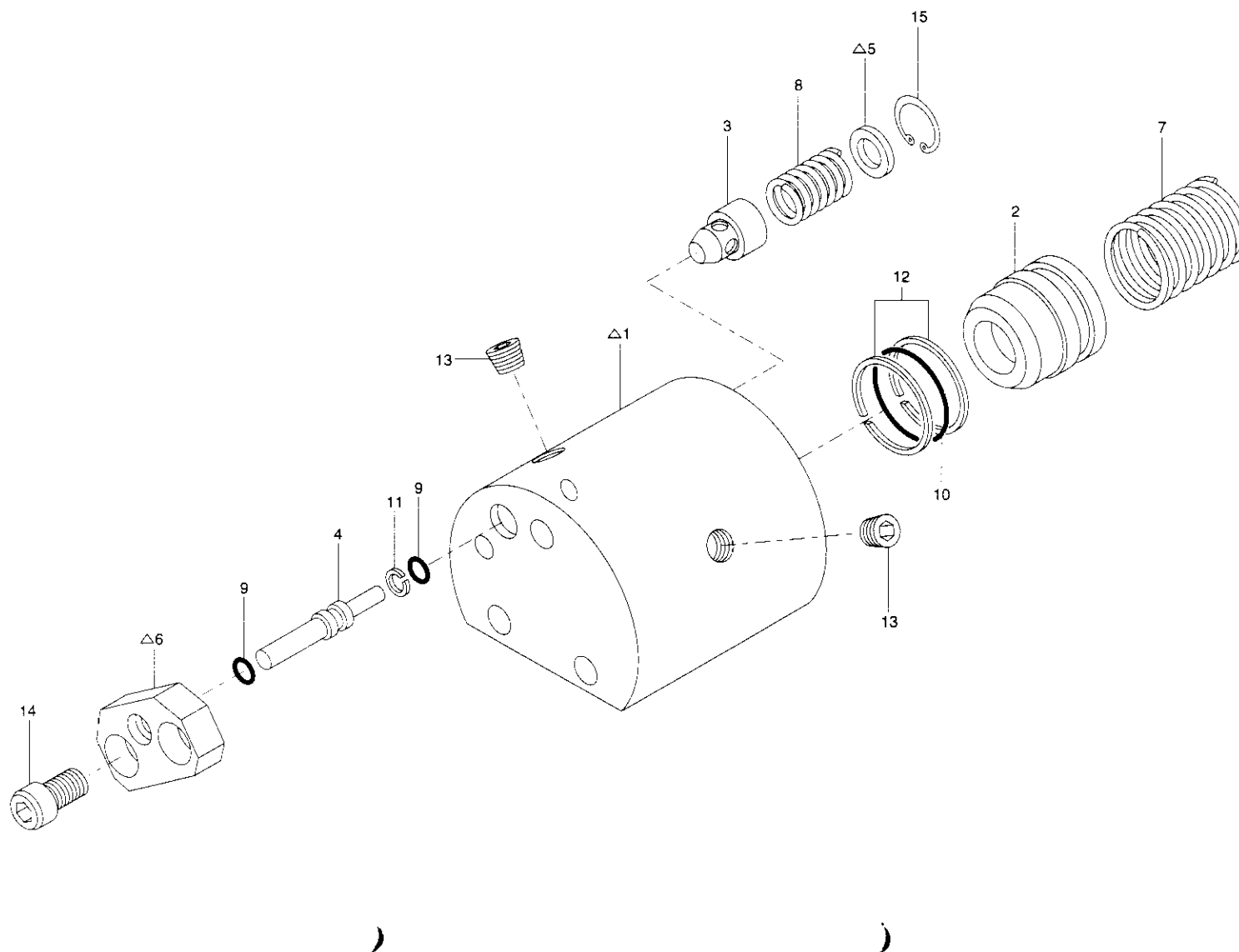
切換バルブ組立(URV374, 375) Fig. 2-4-1 SELECTOR VALVE ASS'Y(URV374, 375)
