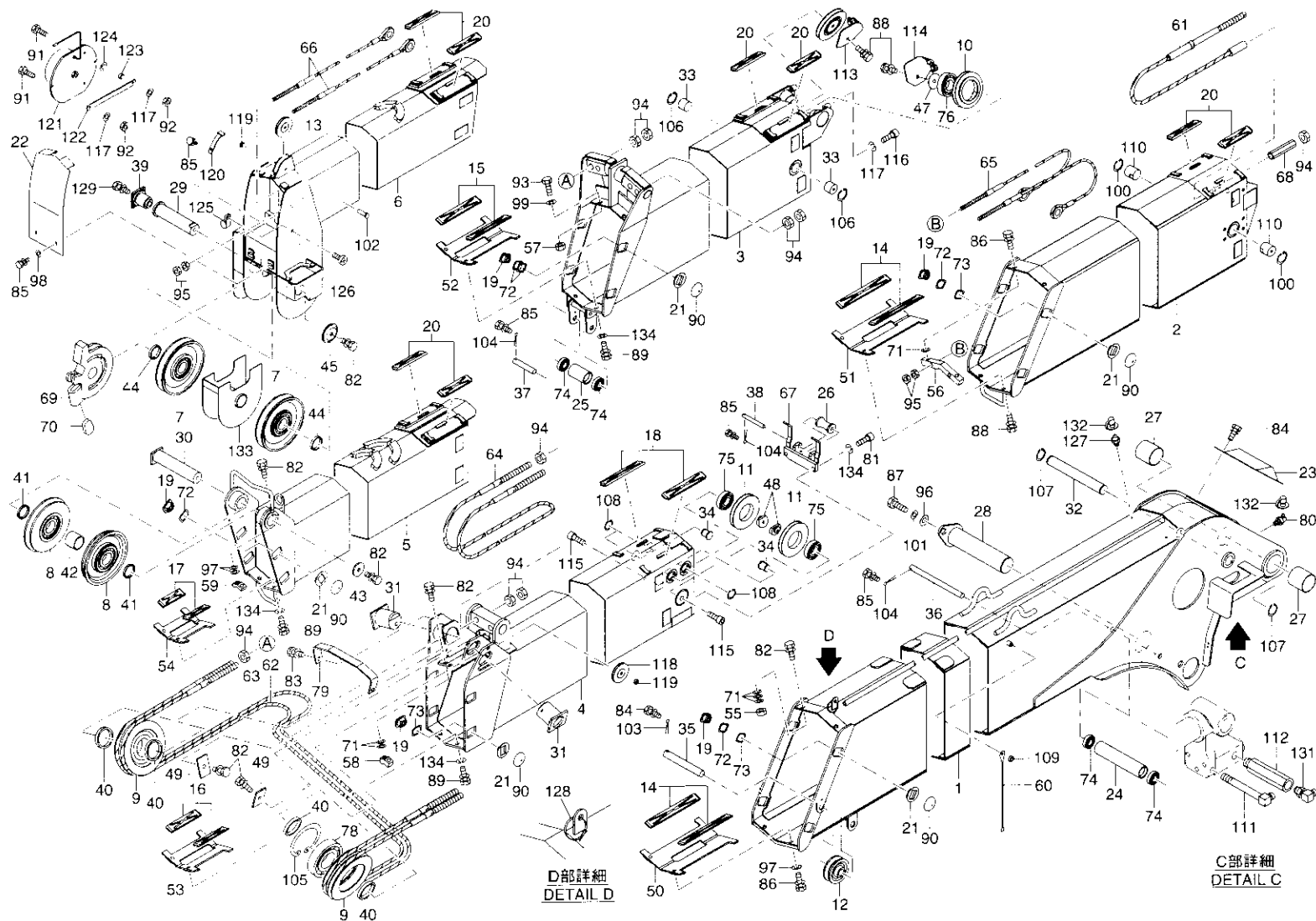
Fig. 1-13 6段ブーム組立(URV376 標準仕様) 6-section BOOM ASS'Y(URV376 STD type)
