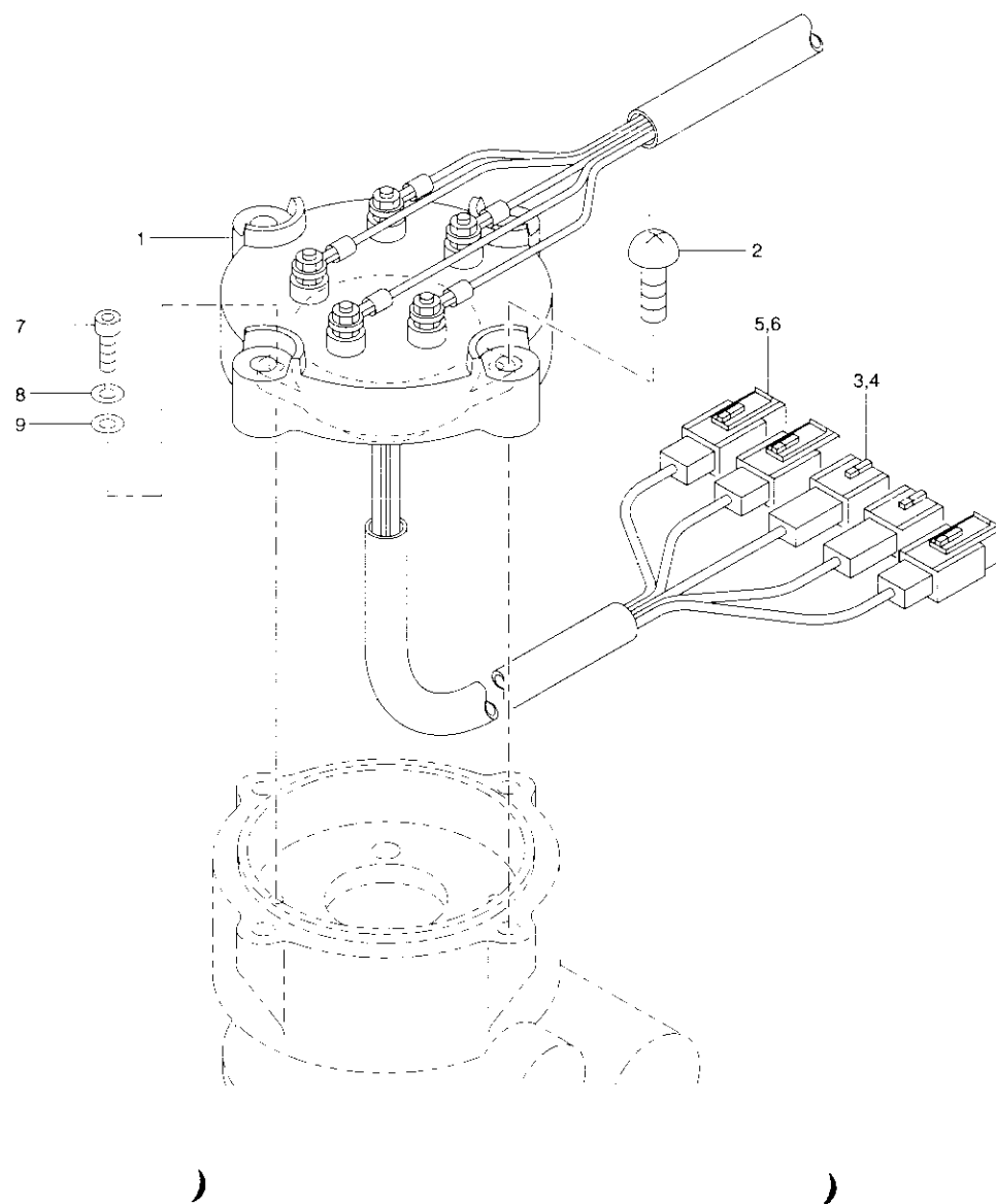
Fig. 13-1-1 スリップリング組立(URV370系 K, 標準仕様) SLIP RING ASS'Y(URV370 series K & STD type)
