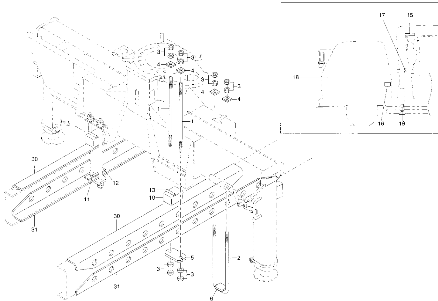
Fig. 25-1 架装組立 MOUNTING ASS'Y
