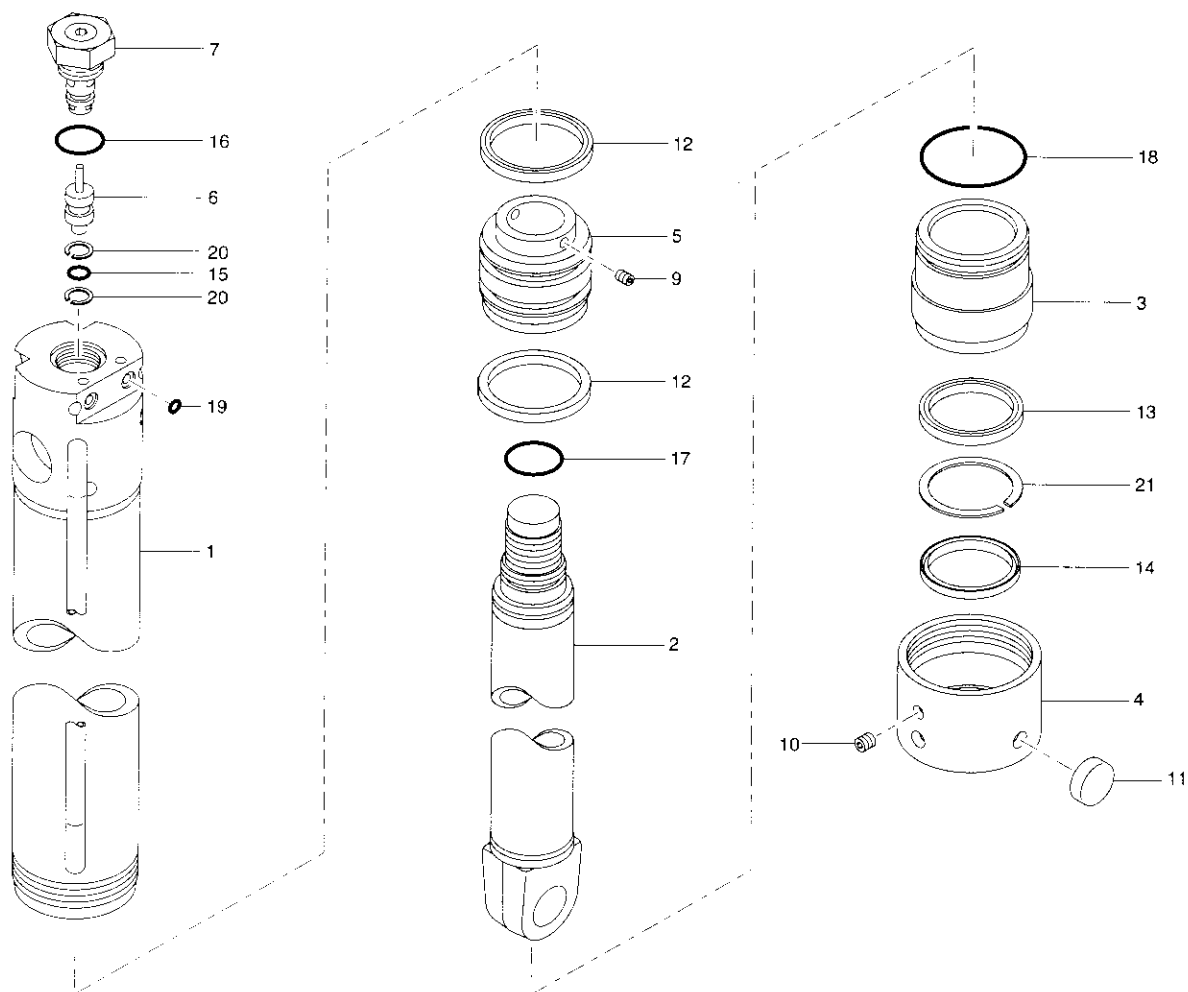
アウトリガシリンダ組立(URV370系 K, 標準仕様) Fig. 12-1 OUTRIGGER CYLINDER ASS'Y(URV370 series K & STD type)
