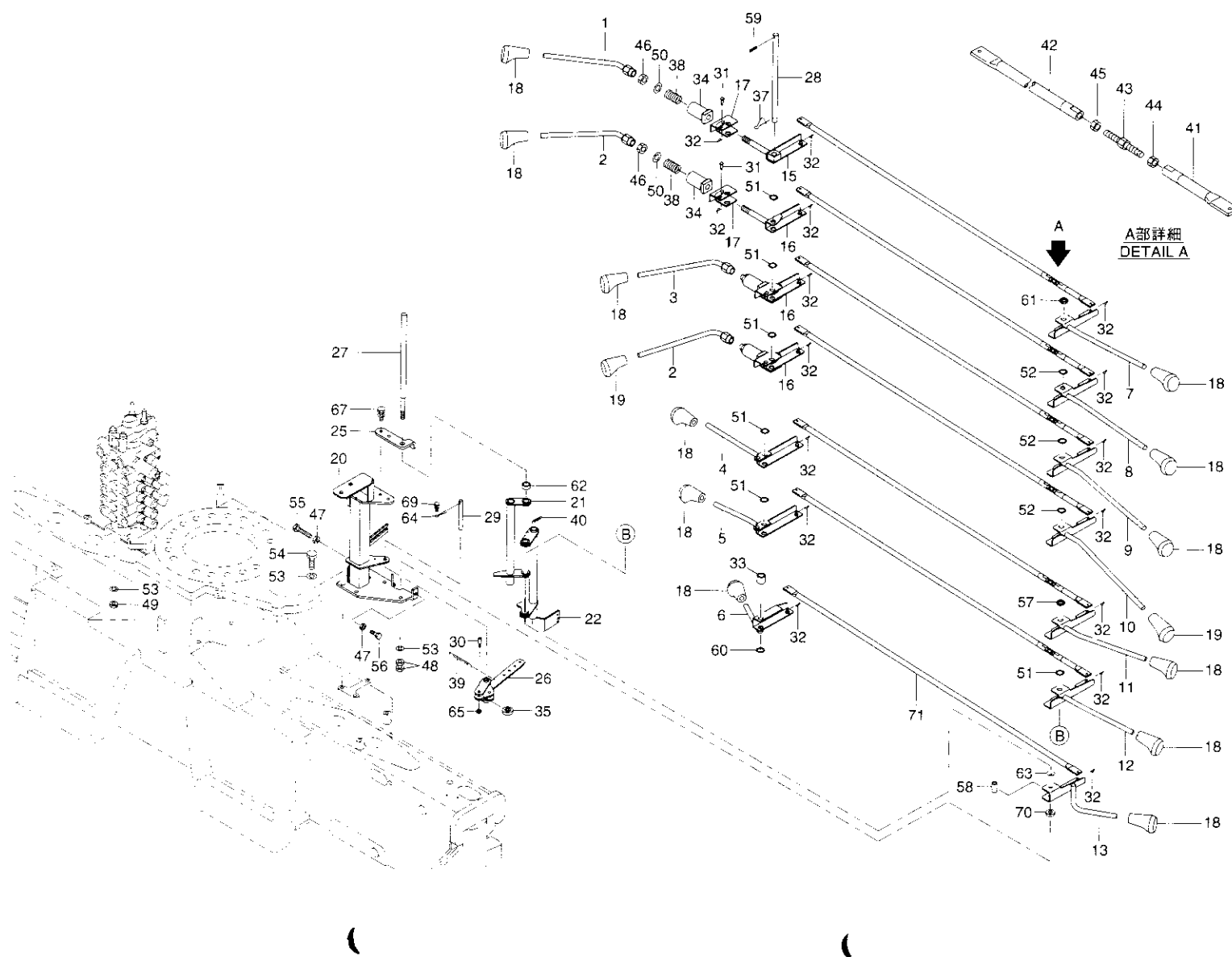
Fig. 14-2 コントロール組立(URV370系 標準仕様) CONTROL ASS'Y(URV370 series STD type)
