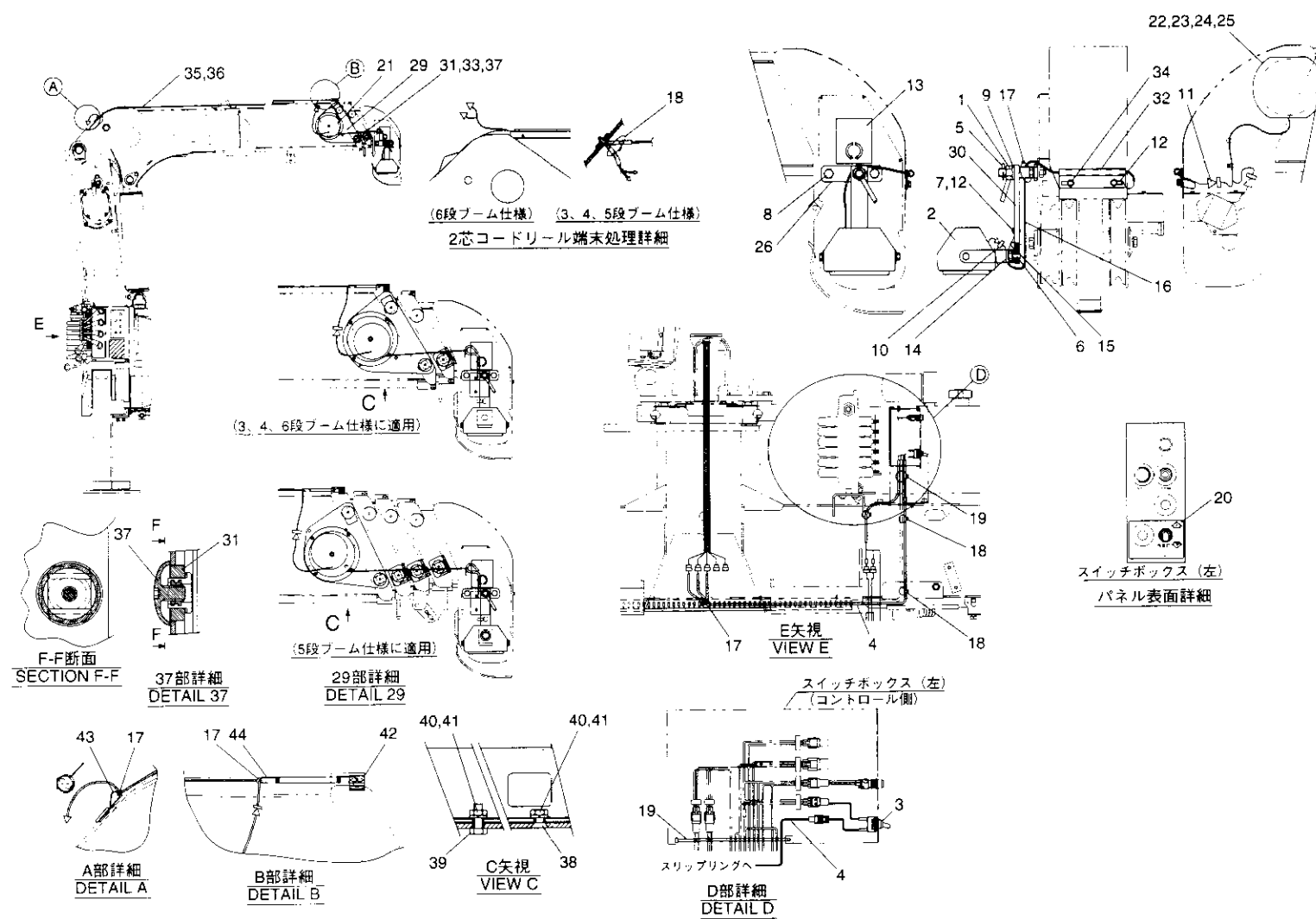
Fig. 30-2 作業灯組立(WL-11)(2芯コードリールタイプ) WORKING LAMP ASS'Y(WL-11)
