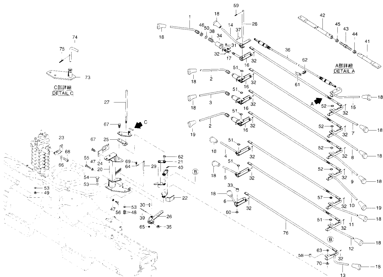
Fig. 14-3 コントロール組立(URV370系 F 仕様) CONTROL ASS'Y(URV370 series F type)
