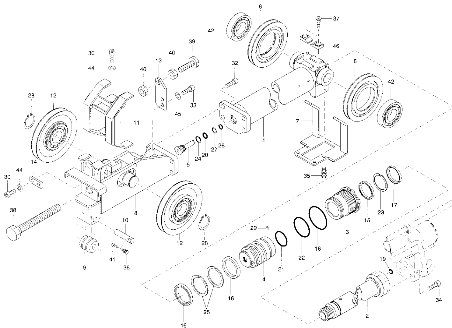
テレスリンダ(2)組立(UKV374) Fig. 2-5 TELESCOPE CYLINDER(2) ASS'Y(UKV374)
