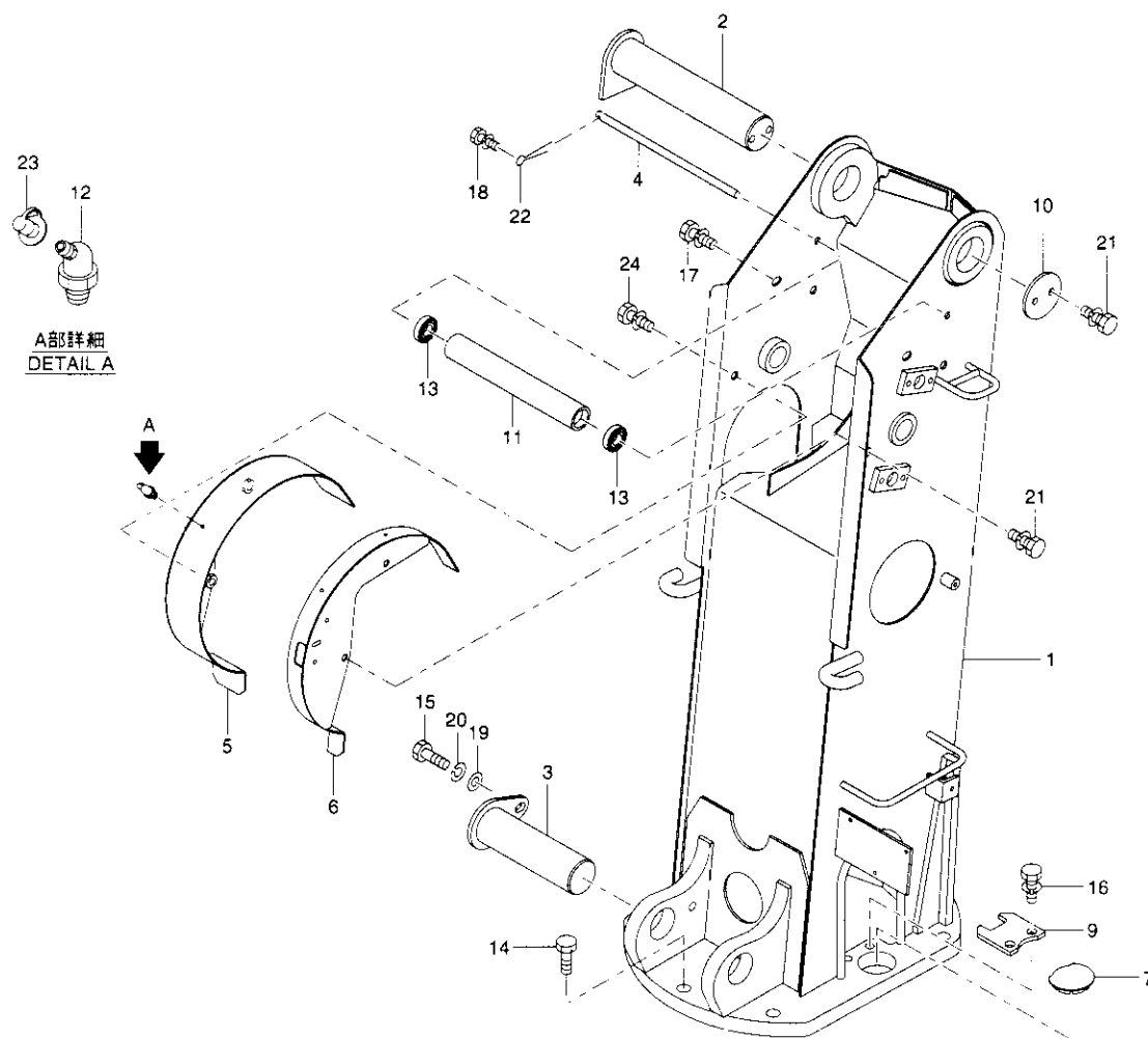
コラム組立(URV370系 F 仕様) Fig. 7-2 COLUMN ASS'Y(URV370 series F type)
