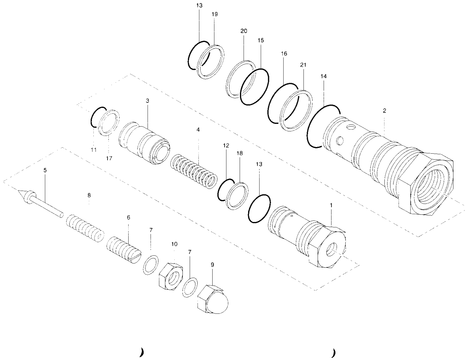
Fig. 24-1-1 リリーフバルブ組立(RT-04A) RELIFE VALVE ASS'Y(RT-04A)
