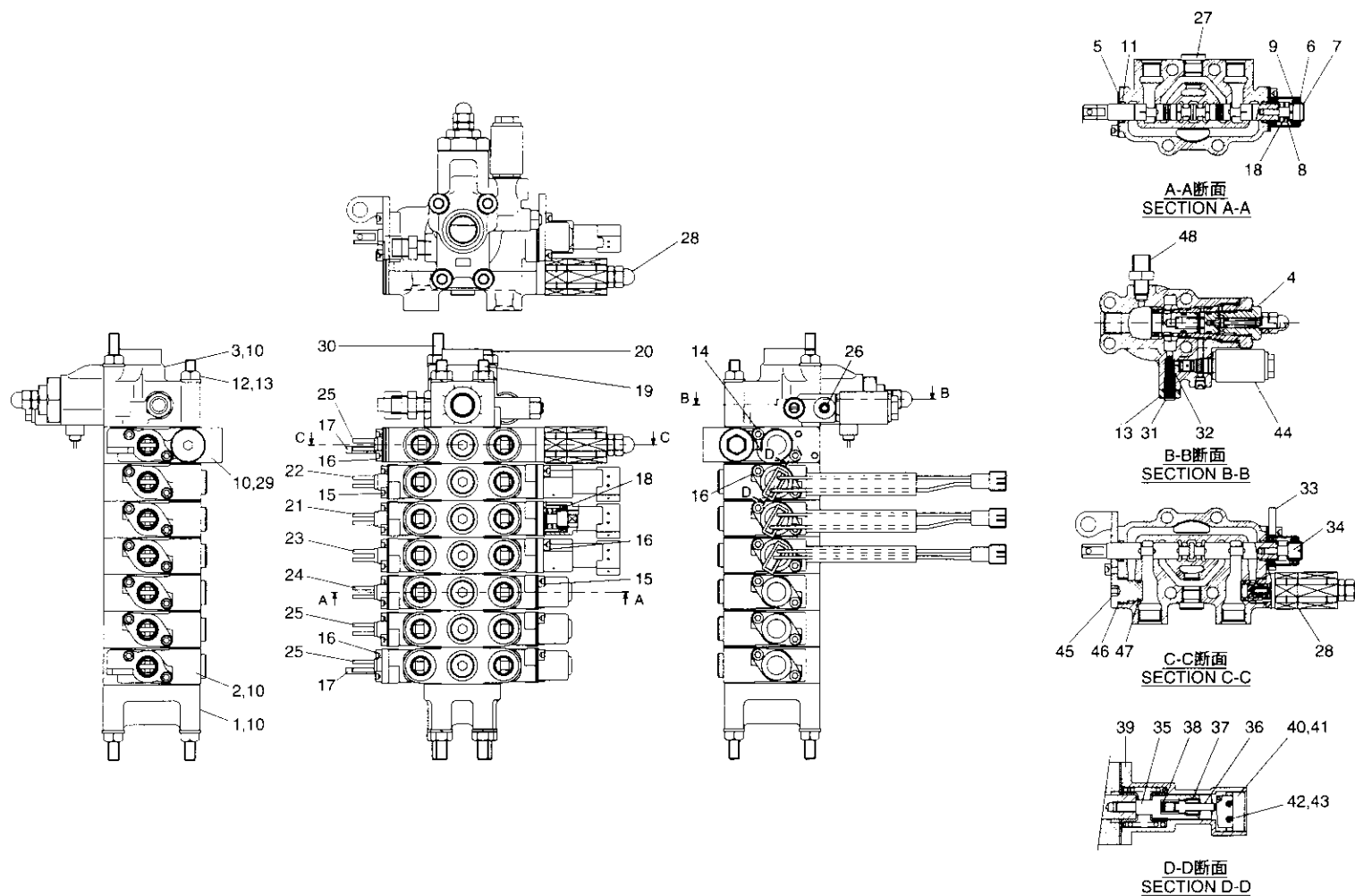
Fig. 24-1 コントロールバルブ組立(7連)(K仕様) CONTROL VALVE ASS'Y(7-spools)(K type)
