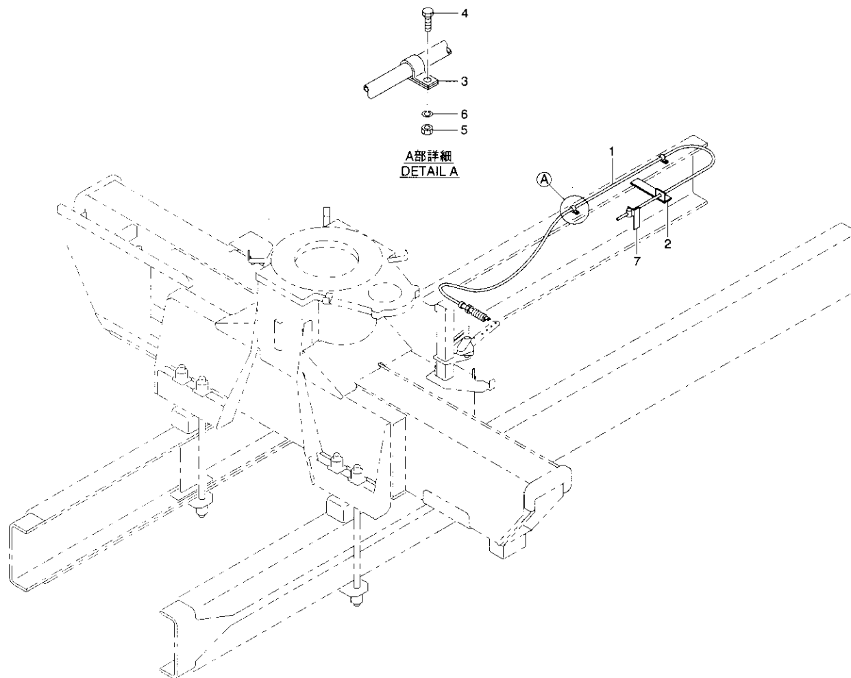
Fig. 25-2 アクセルコントロール組立 ACCELERATOR CONTROL ASS'Y
