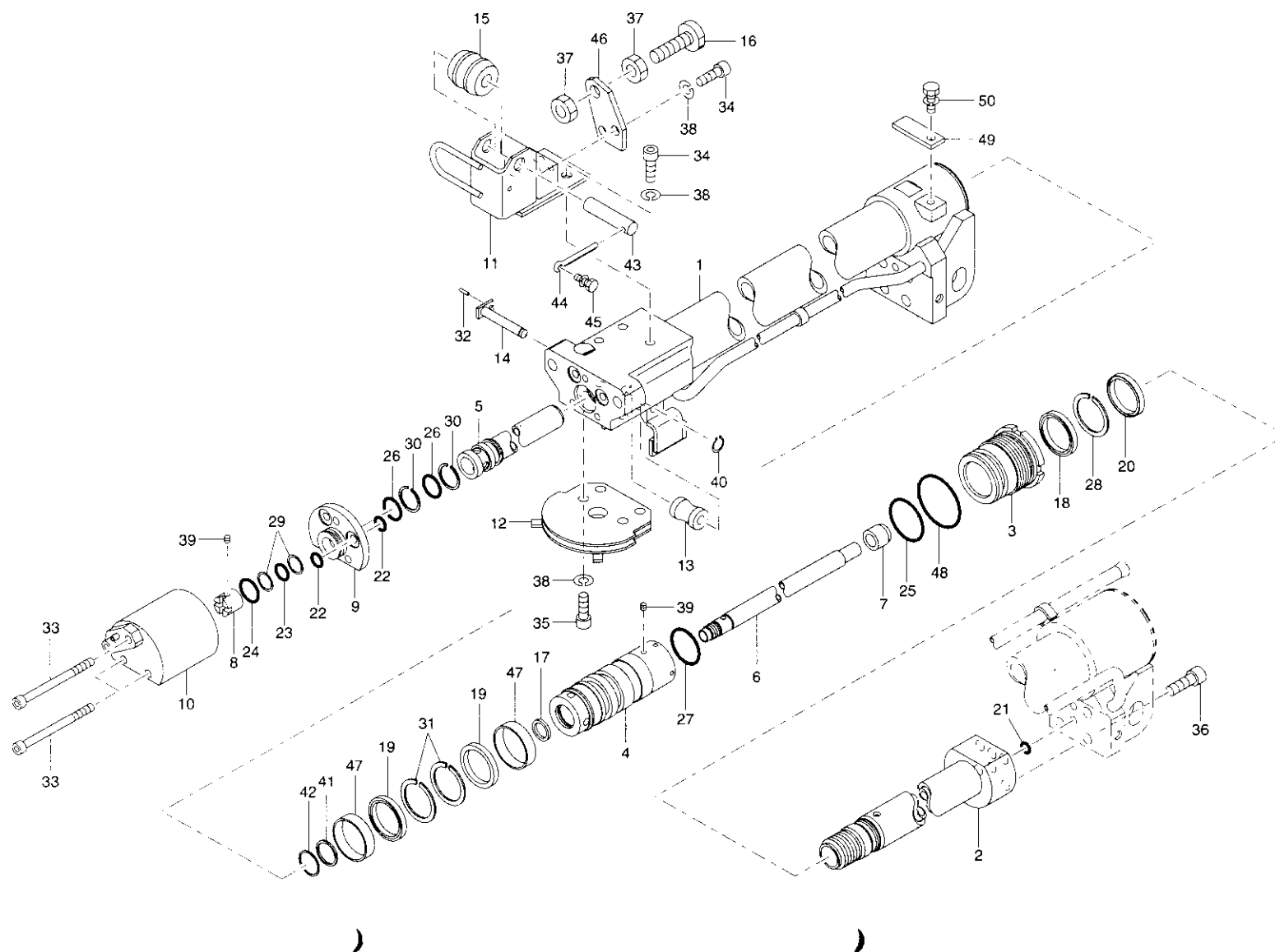
テレシリンダ(2)組立(UKV375) Fig. 2-7 TELESCOPE CYLINDER(2) ASS'Y(UKV375)
