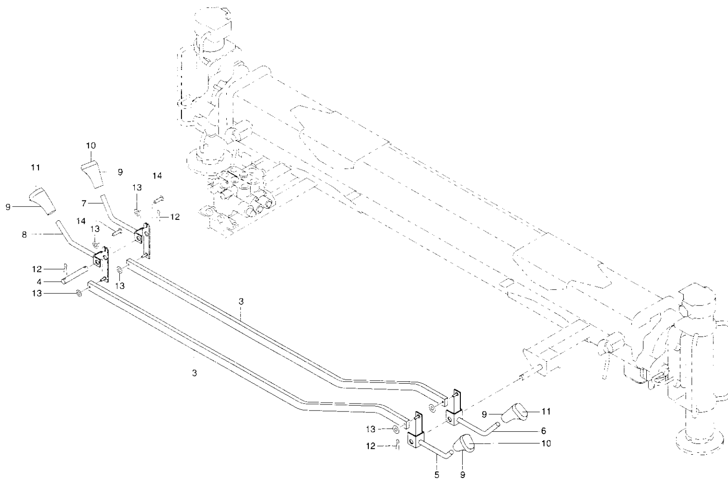
Fig. 20-4 コントロール (リヤアウト) 組立 (URV376) CONTROL (Rear outrigger) ASS'Y (URV376)
