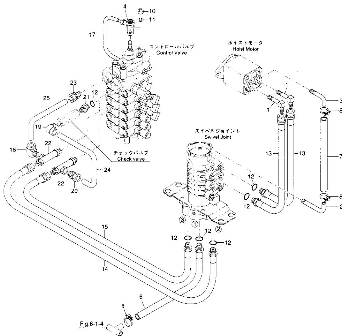
パイピング(ホイストモータ)(URV370系 K 仕様) Fig. 6-1-2 PIPING(Hoist motor)(URV370 series K type)
