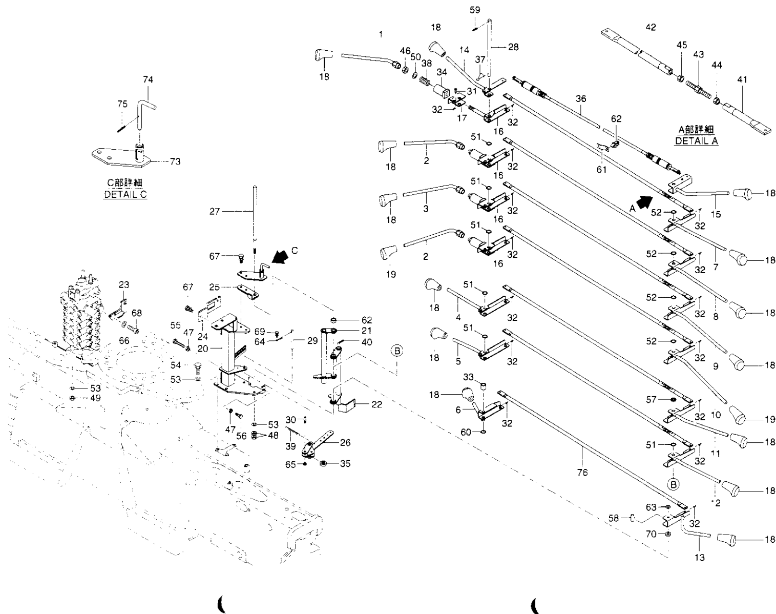
コントロール組立(URV370系 F 仕様) Fig. 14-3 CONTROL ASS'Y(URV370 series F type)
