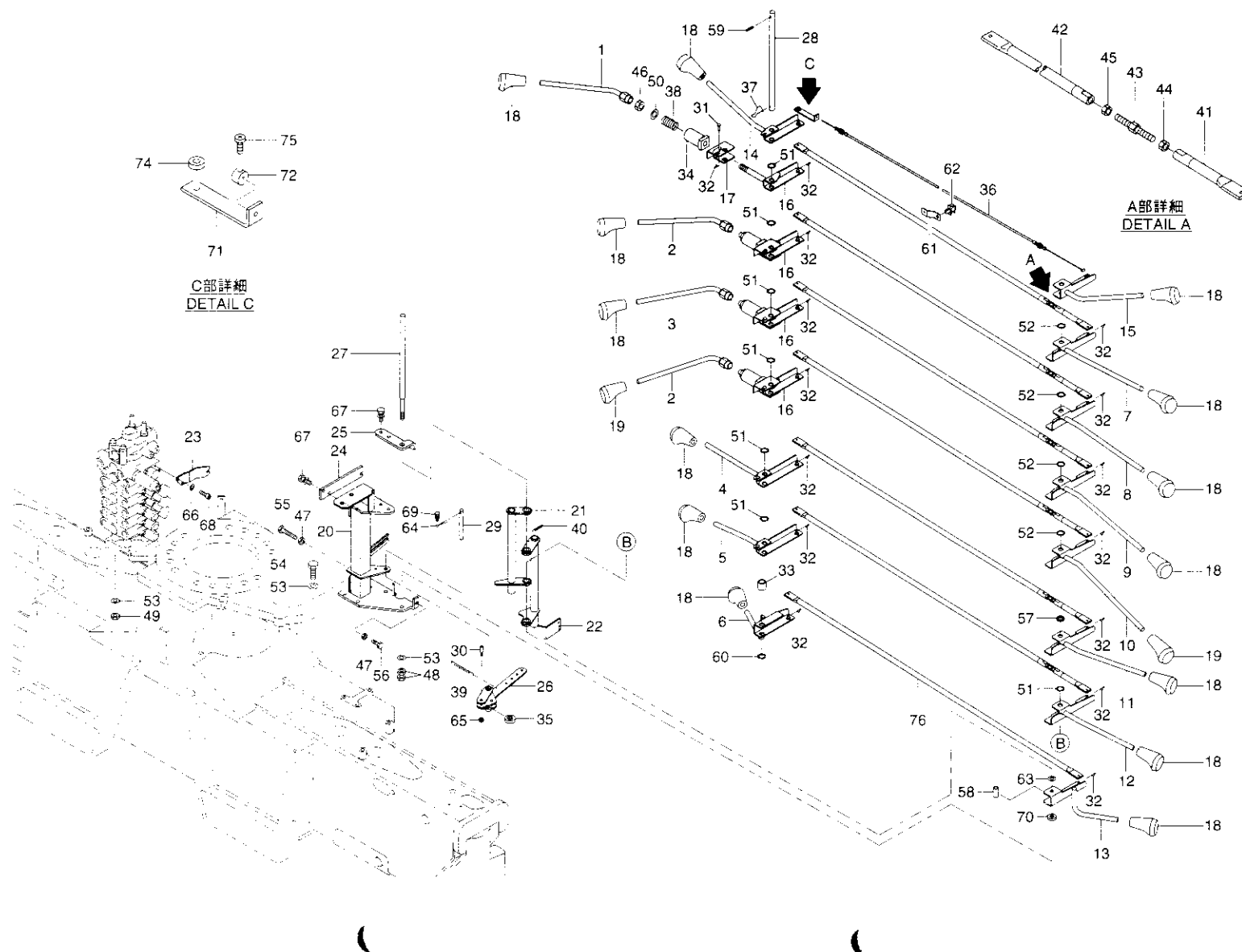
コントロール組立(URV370系 K 仕様) Fig. 14-1 CONTROL ASS'Y(URV370 series K type)
