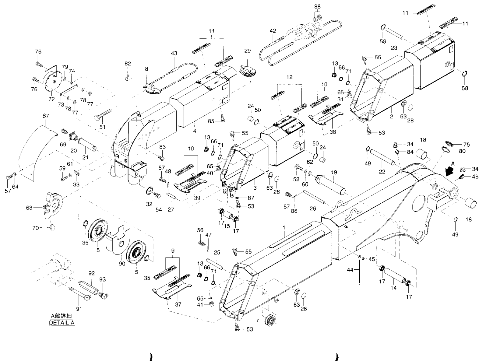
Fig. 1-8 4段ブーム組立(URV374 標準仕様) 4-section BOOM ASS'Y(URV374 STD type)
