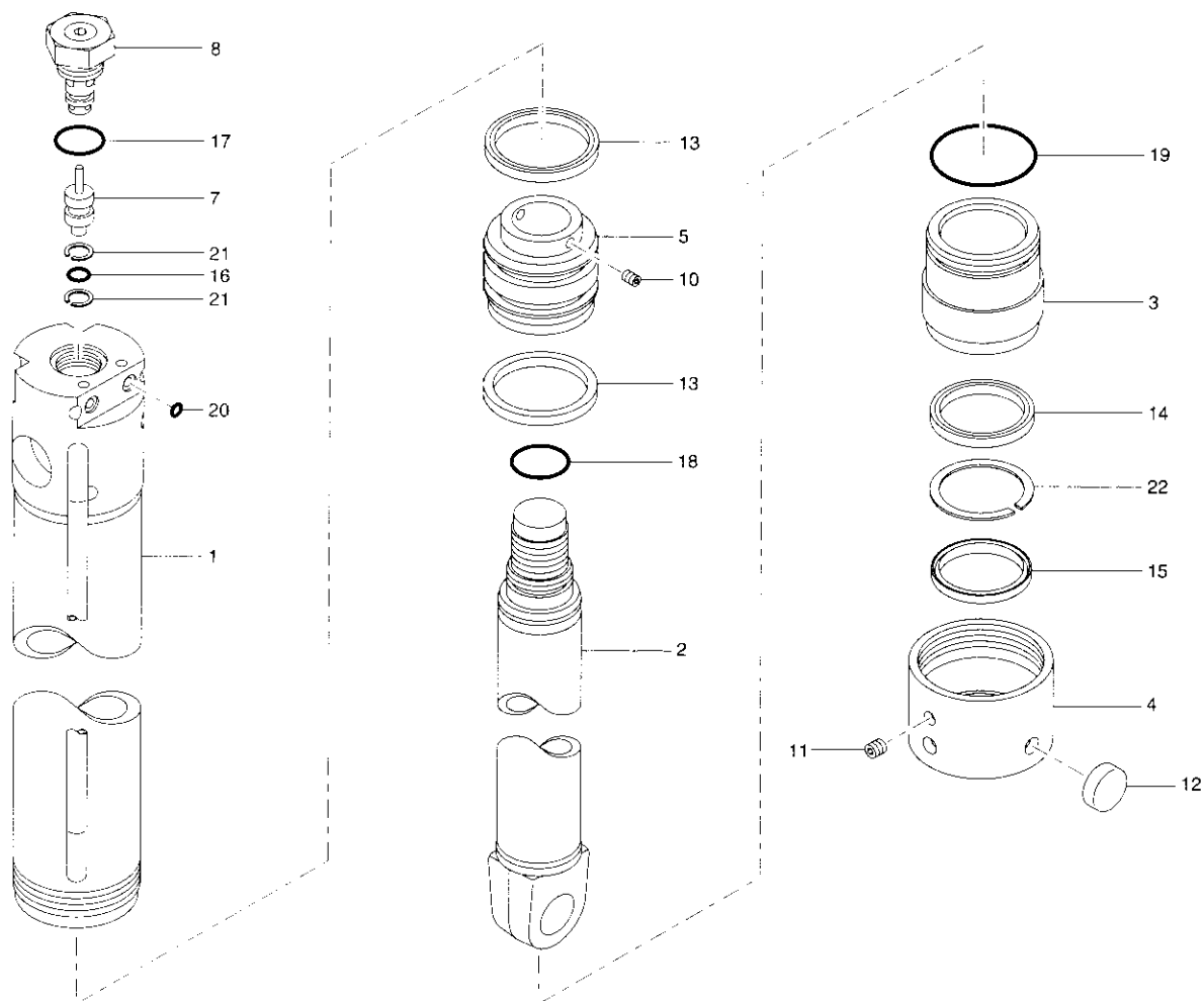
アウトリガシリンダ組立(URV370系 GK, G 仕様) Fig. 12-2 OUTRIGGER CYLINDER ASS'Y(URV370 series GK & G type)
