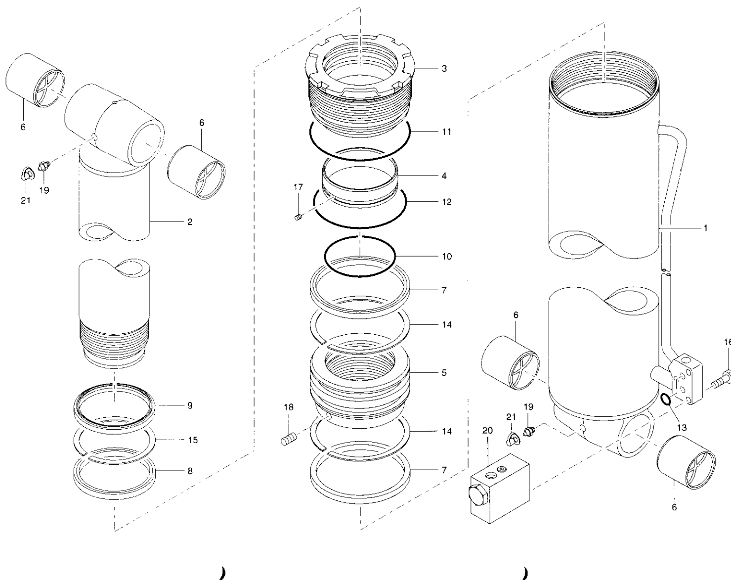
Fig. 11-1 Derrick Cylinder Ass'y (ALL MODELS) デリックシリンダ組立(全機種共通)
