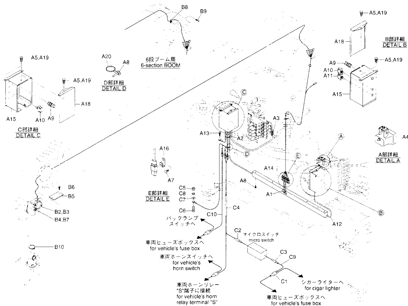
警報装置組立(URV370系 RK, R 仕様)
