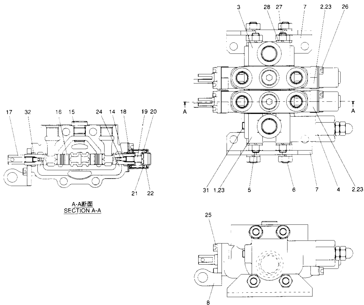
Fig. 24-6 コントロールバルブ組立(2連)(リヤアウトリガ) CONTROL VALVE ASS'Y(2-spools)(Rear outrigger)
