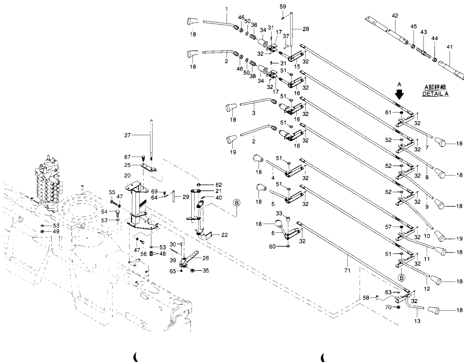
コントロール組立(URV370系 標準仕様) Fig. 14-2 CONTROL ASS'Y(URV370 series STD type)
