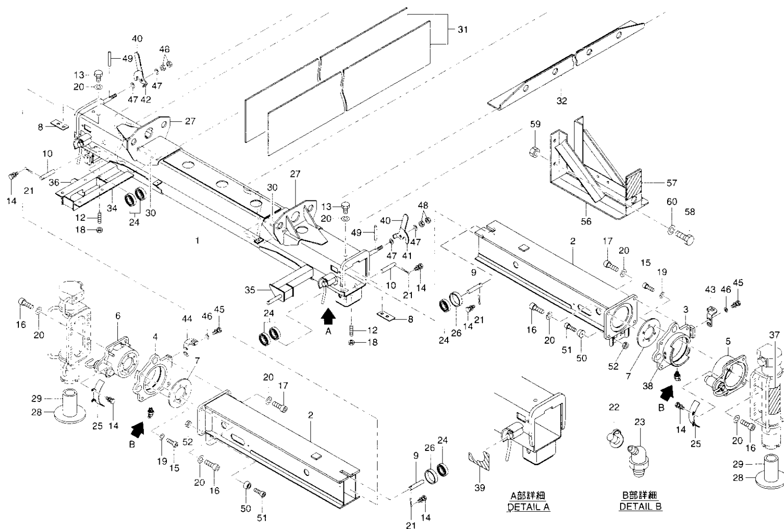
Fig. 20-1 リヤアウトリガ組立 (URV376) REAR OUTRIGGER ASS'Y (URV376)
