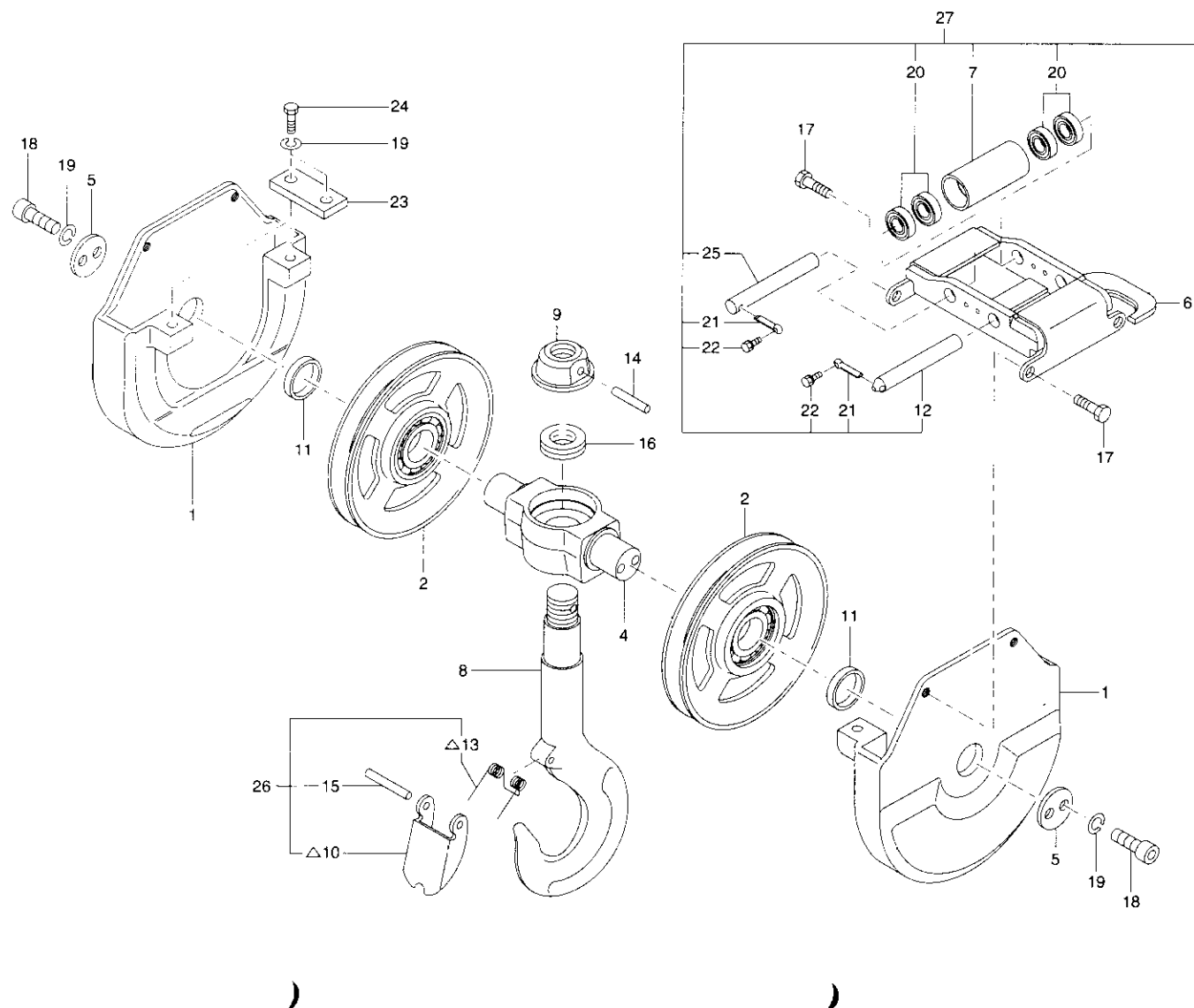
フック組立(URV370系 K 仕様) Fig. 3-1 HOOK ASS'Y(URV370 series K type)
