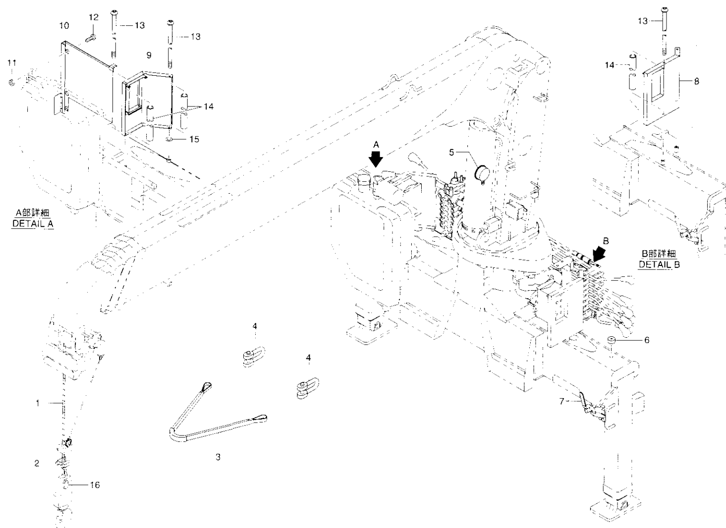
Fig. 17-3-1 装備品(1)(URV370系 F 仕様) EQUIPMENT(1)(URV370 series F type)
