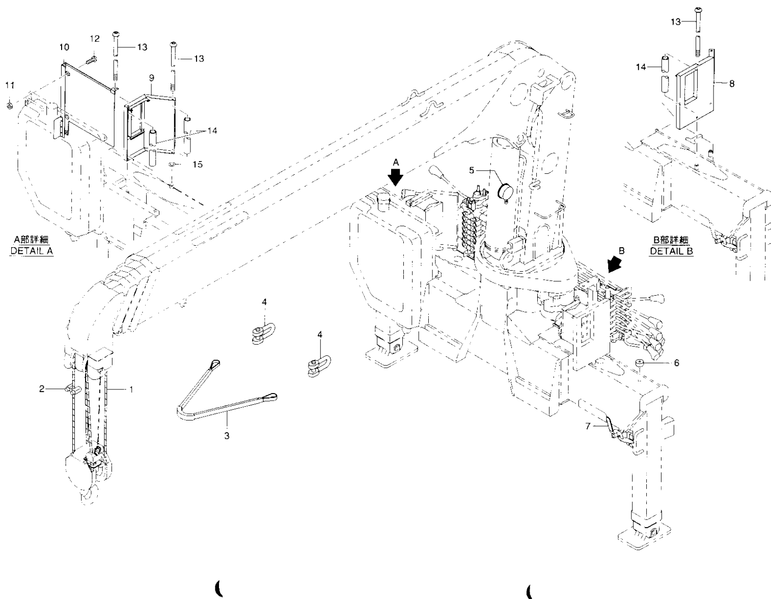
Fig. 17-1-1 装備品(1)(URV370系 K 仕様) EQUIPMENT(1)(URV370 series K type)
