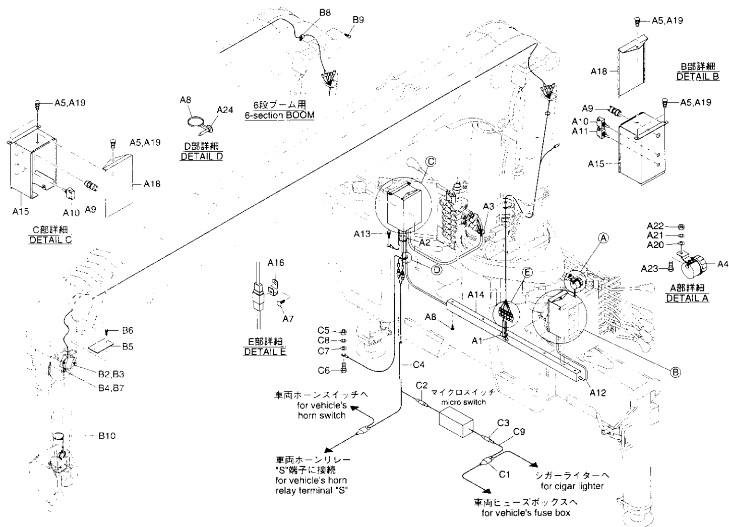
警報装置組立(URV370系 K 仕様) Fig. 4-1 ALARM DEVICE ASS'Y(URV370 series K type)
