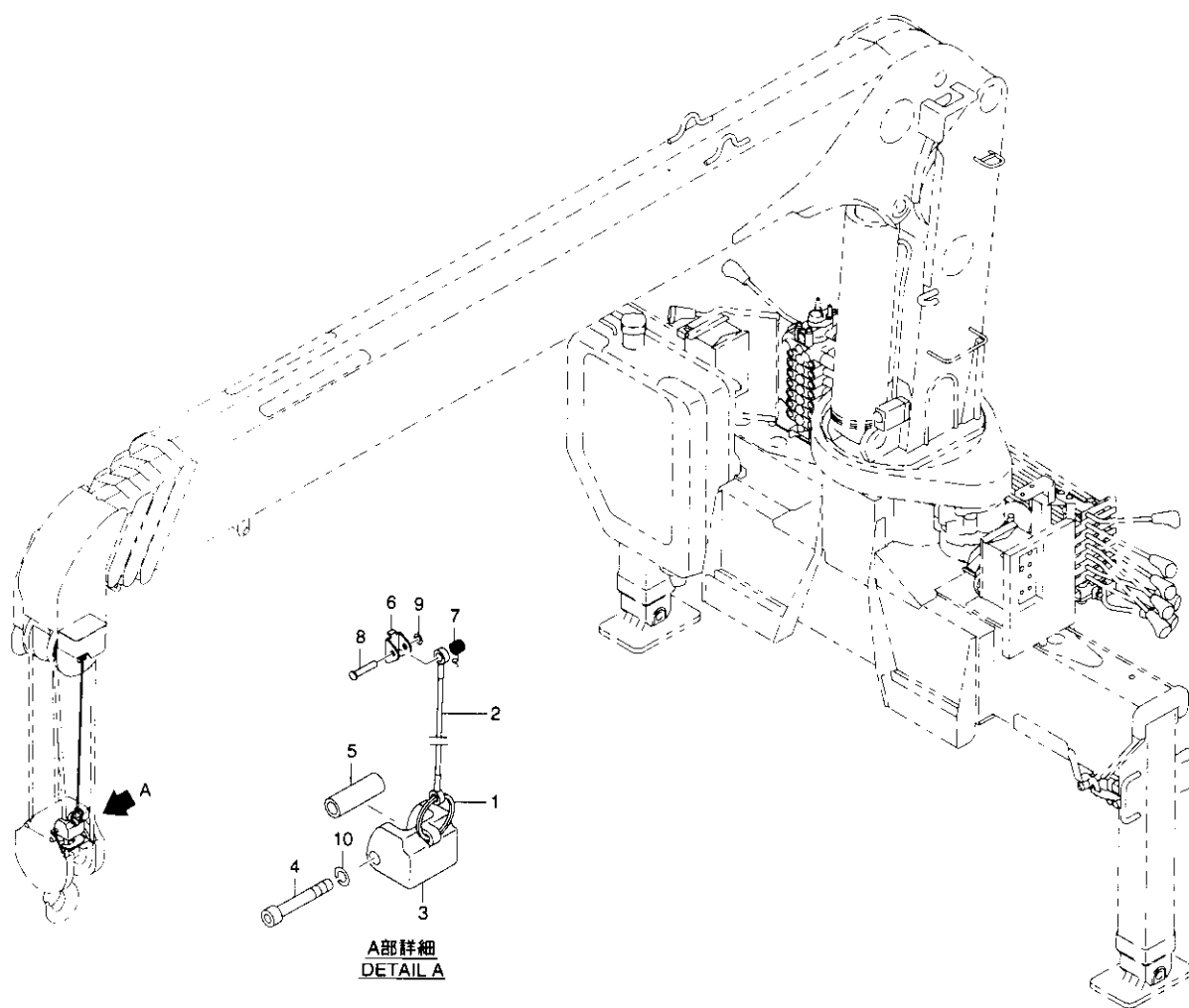
Fig. 17-1-2 装備品(2)(URV370系 K 仕様) EQUIPMENT(2)(URV370 series K type)
