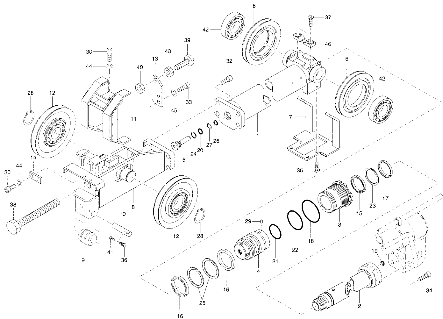
テレシリンダ(2)組立(URV374) Fig. 2-5 TELESCOPE CYLINDER(2) ASS'Y(URV374)
