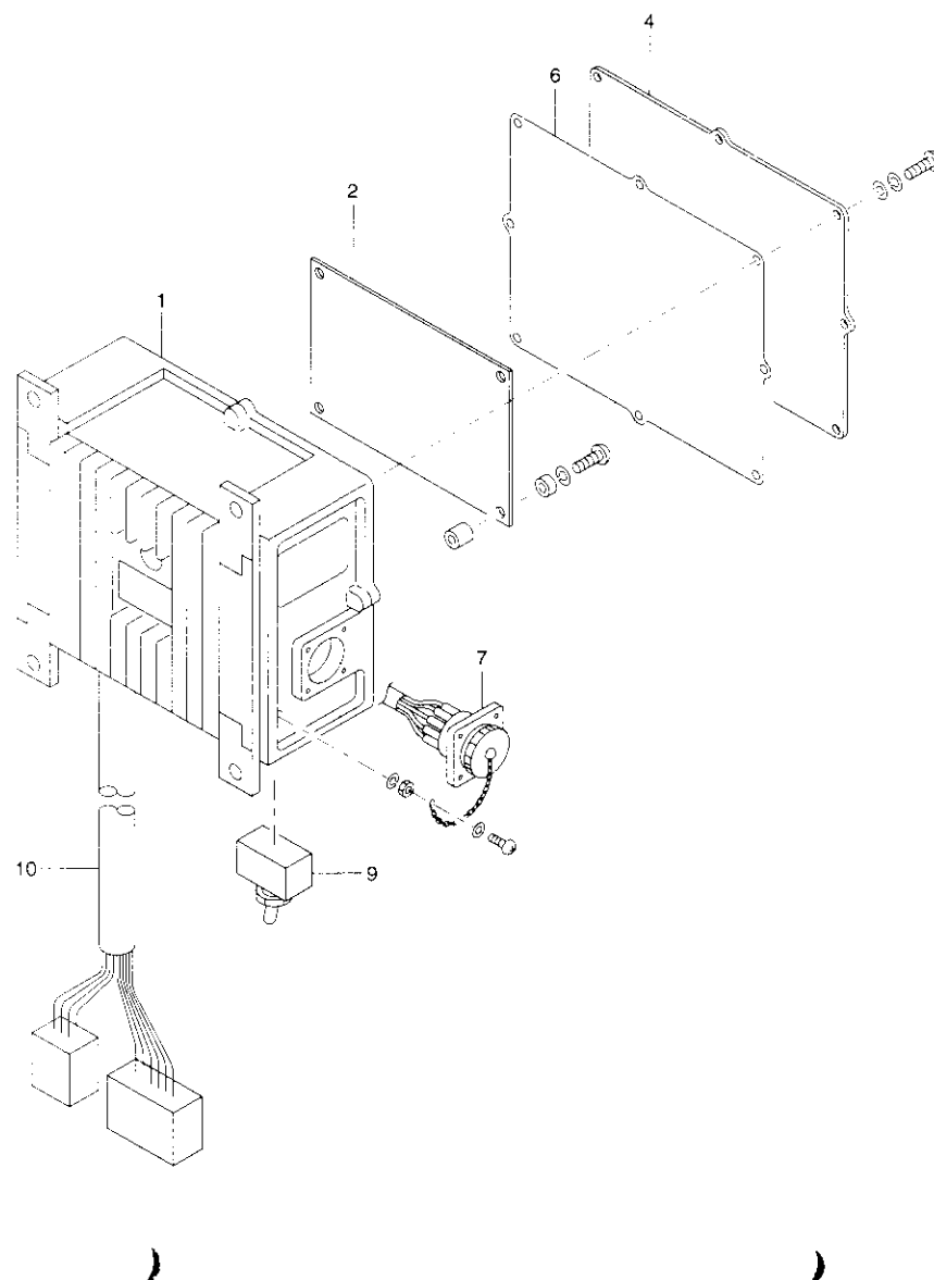
Fig. 21-1-1 コントロールボックス組立 (URV370系 RK, R 仕様) CONTROL BOX ASS'Y (URV370 series RK & R type)
