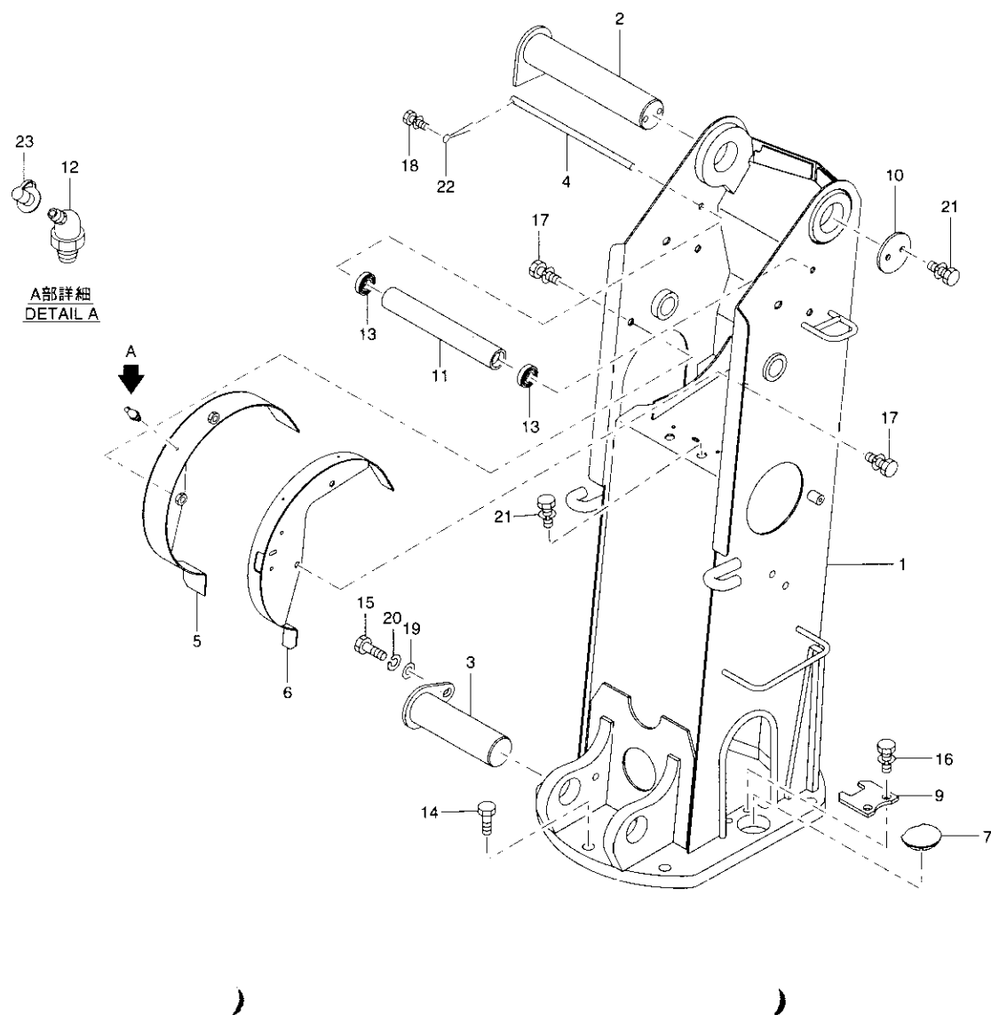
コラム組立(URV370系 K, 標準仕様) Fig. 7-1 COLUMN ASS'Y(URV370 series K & STD type)
