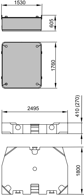
Central ballast · 车体中心配重
