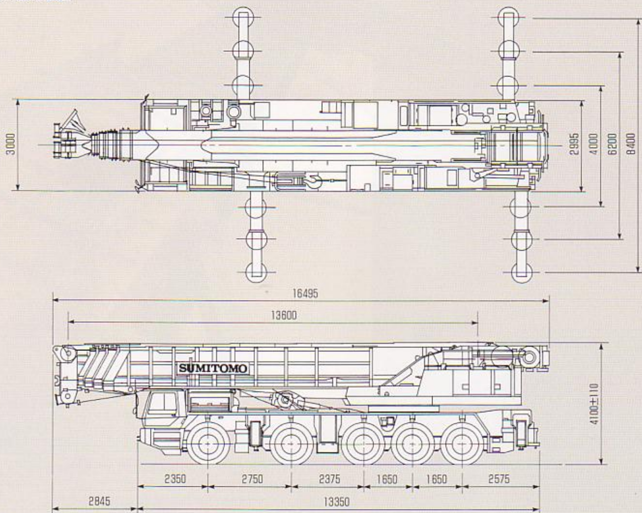
■外観寸法図
