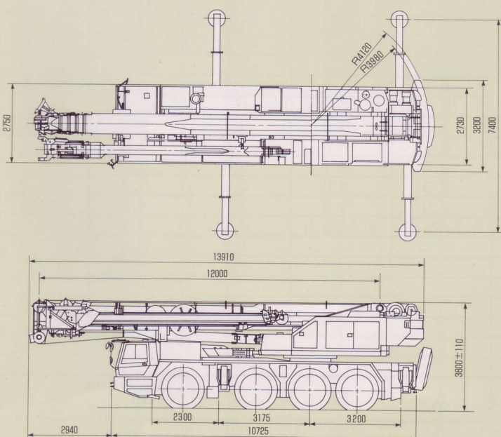
■外観寸法図
