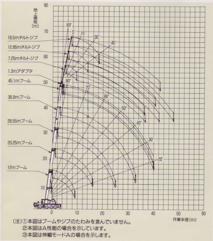
■作業範囲図
