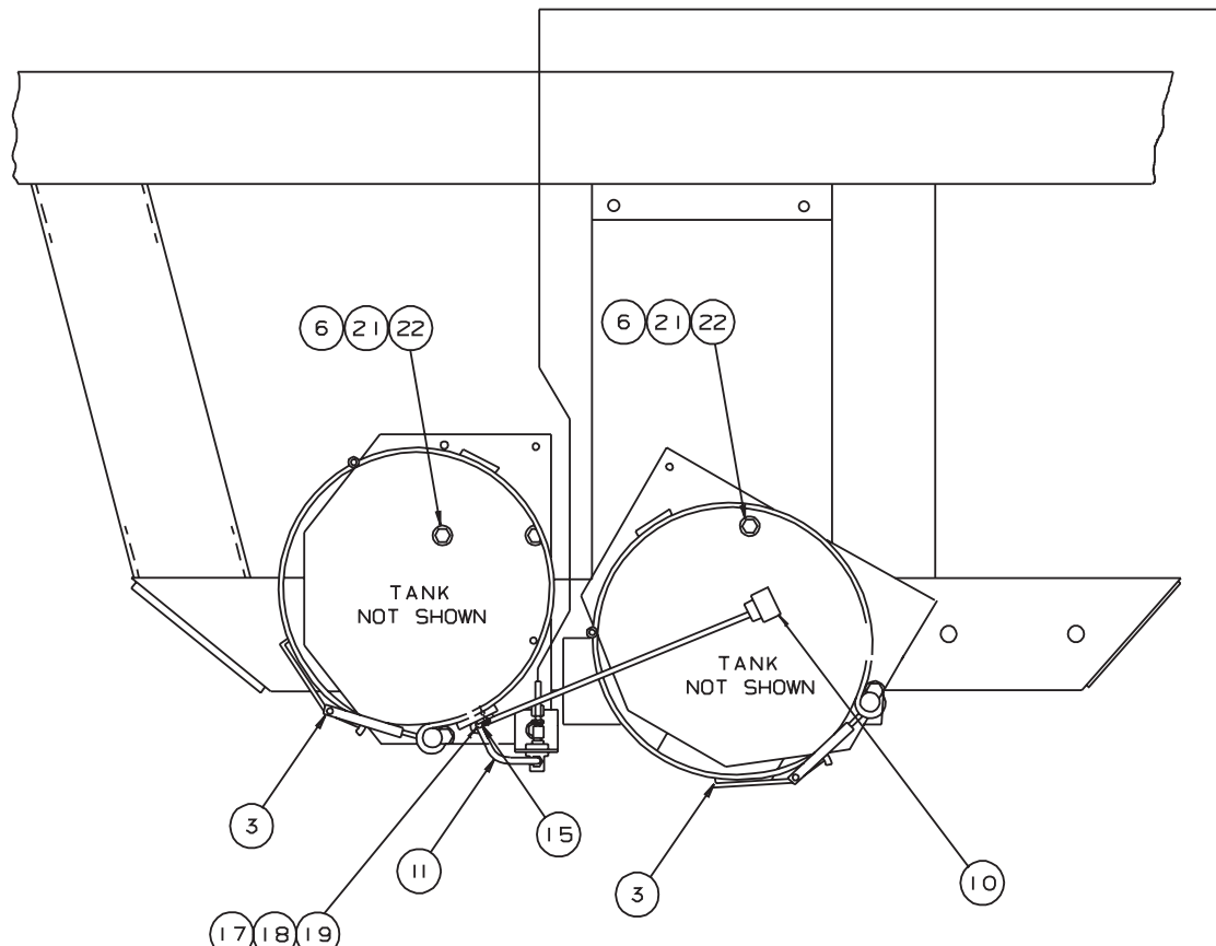
VIEW A-A
