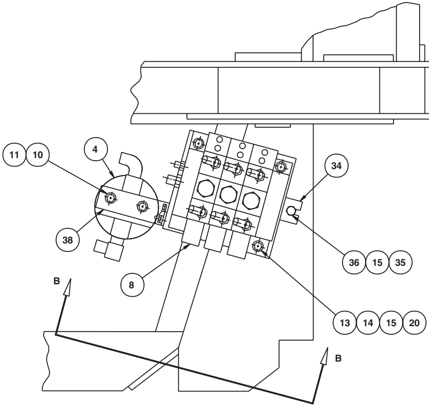
VIEW A-A
