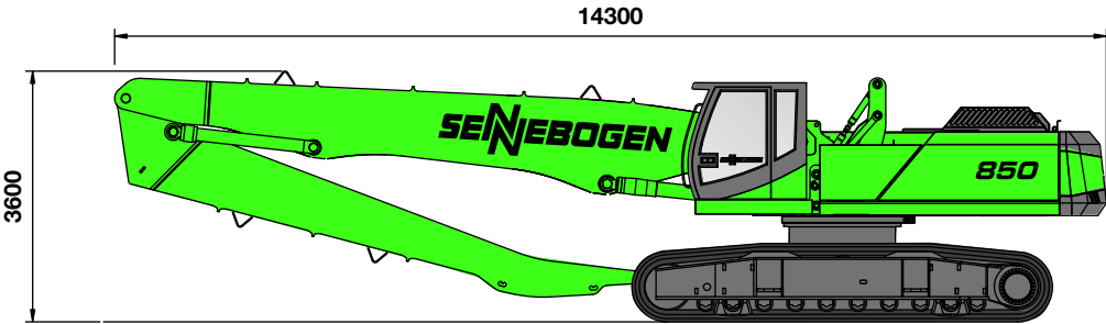
850 R-HD mit Ladeausleger 9,7 m und Greiferstiel 7,8 m 850 R-HD with Loading boom 9.7 m and Grabstick 7.8 m
