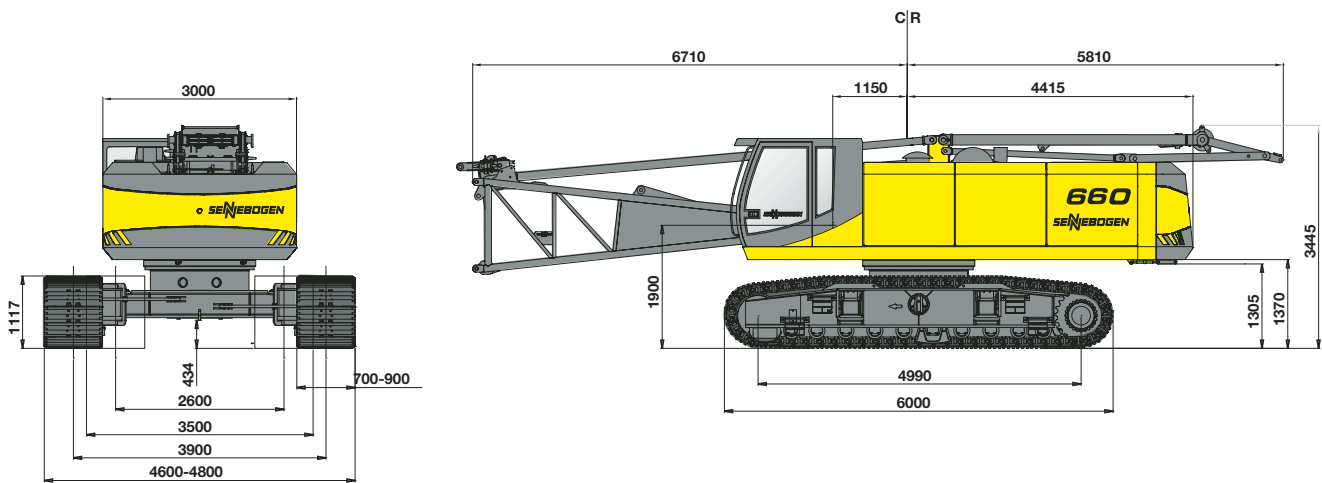
660 HD mit Raupenlaufwerk B7, Länge 6000 mm - 660 HD with crawler B7, length 6000 mm
