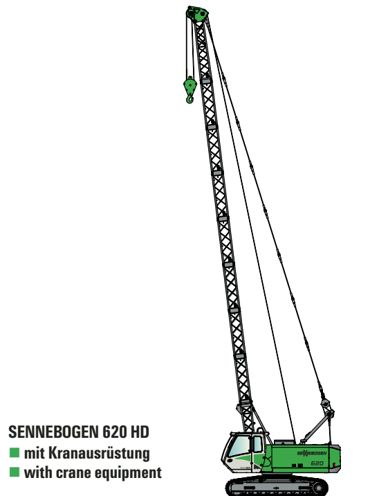
SENNEBOGEN 620 HD ■ mit Verrohrungs­maschine und Bohrgreifer ■ with casing oscillator and pilegrab
