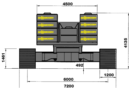
mit Laufwerk B9HD 8800 mm Länge - with crawler B9HD 8800 mm length
