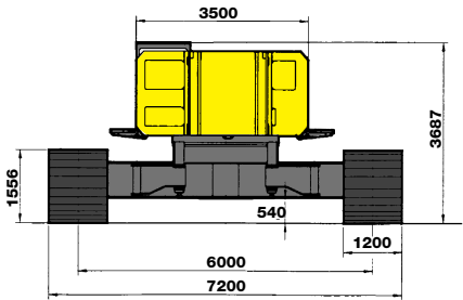
mit Laufwerk B10S 8800 mm Länge - with crawler B10S 8800 mm length
