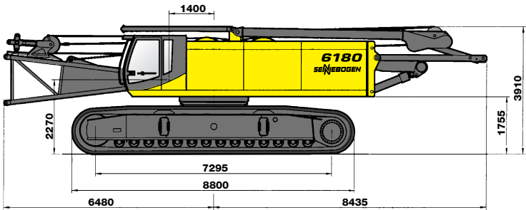
mit Laufwerk B9HD 8800 mm Länge - with crawler B9HD 8800 mm length
