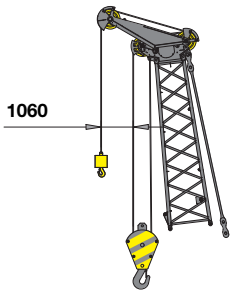
Hauptausleger SHLH mit Schnabelausleger S12.1(12t) Main boom SHLH with Auxiliary jib S12.1(12t)
