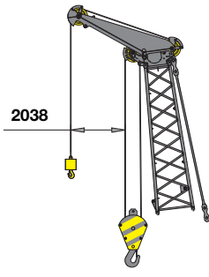
Hauptausleger SH mit Schnabelausleger S24.1(24t) Main boom SH with Auxiliary jib S24.1(24t)
