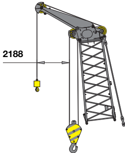
Hauptausleger SHLH mit Schnabelausleger S24.1(24t) Main boom SHLH with Auxiliary jib S24.1(24t)
