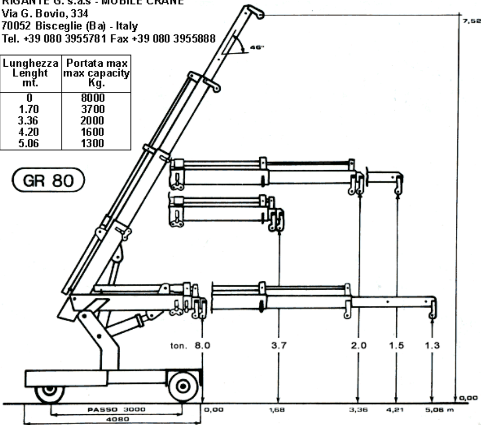
Diagramma portate Test-chart GR 80
