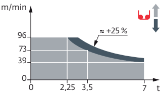
75 LVF 35 Optima
