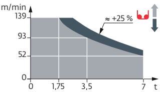
100 LVF 35 Optima
