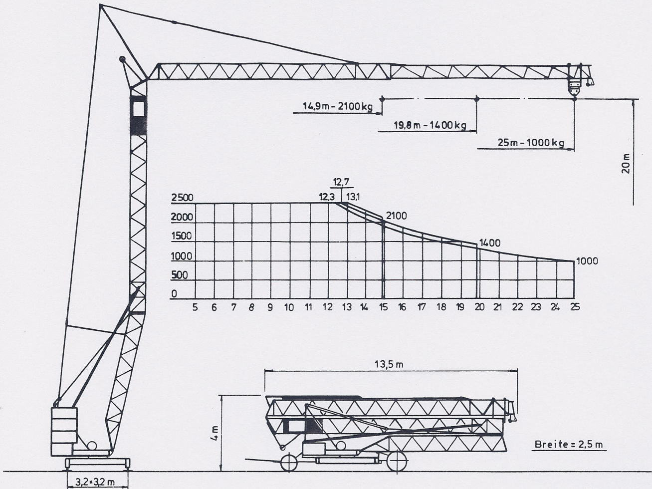
Turmdrehkran mit Teleskopausleger
