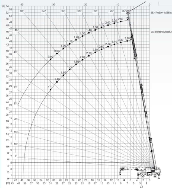
FLY - Stabilizzatori completamente estesi FLY - Outriggers full extended
