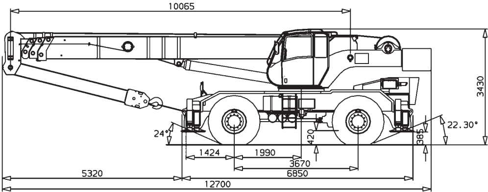
Dimensioni (mm)
