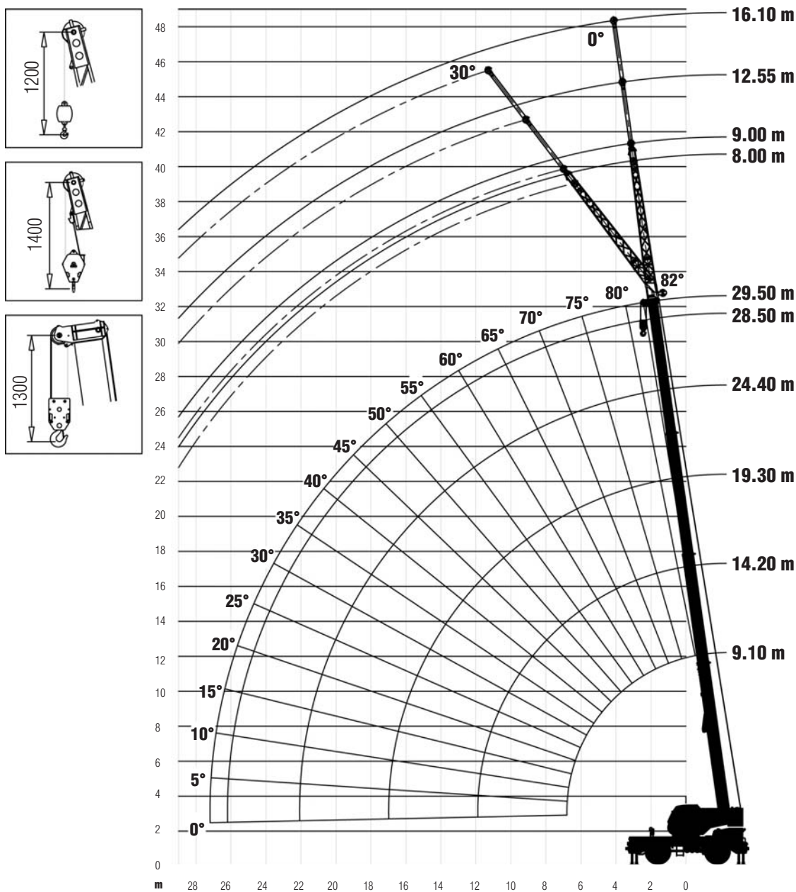
DIAGRAMMA DI LAVORO - WORKING DIAGRAM - DIAGRAMME DE TRAVAIL - ARBEITSBEREICH - DIAGRAMA DE TRABAJO
