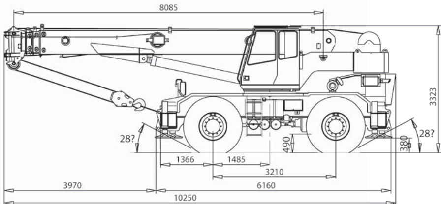
Dimensioni (mm)
