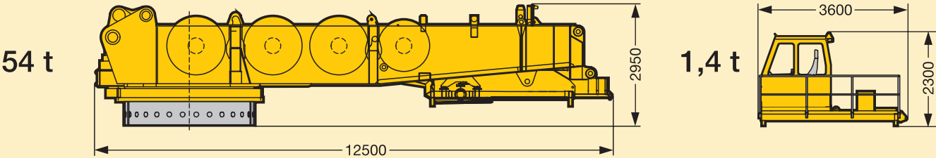
Querträger / Lateral beam / Poutre transversale
