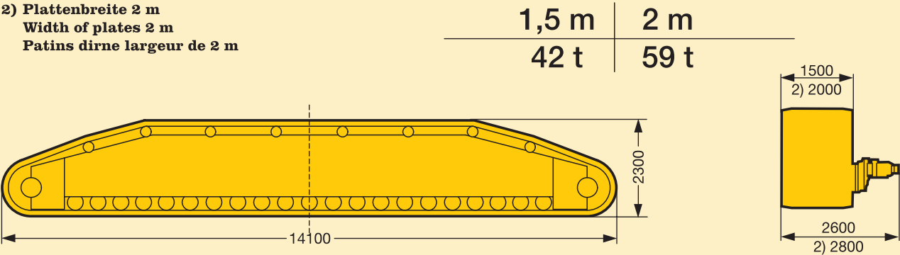
Raupenträger / Crawler carrier / Porteur chenilles
