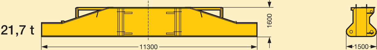
Raupenmittelteil / Crawler center frame / Partie centrale
