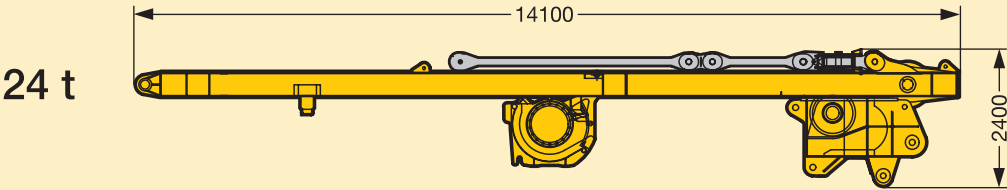
Raupenmittelteil / Crawler center frame / Partie centrale
