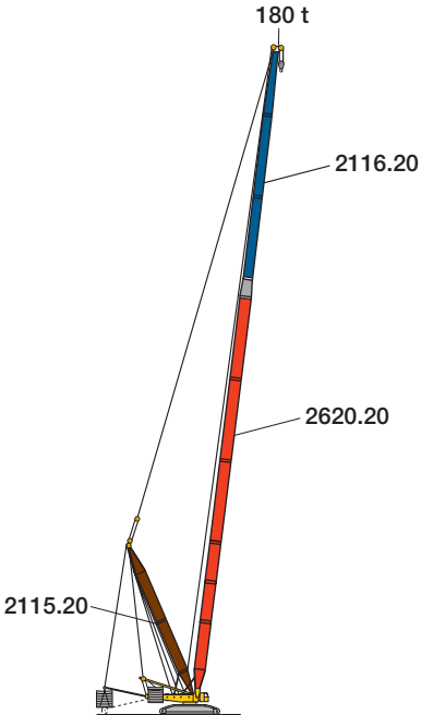
SwD/SwDB/BW Sw 35 m – 112 m D 21 m – 28 m
