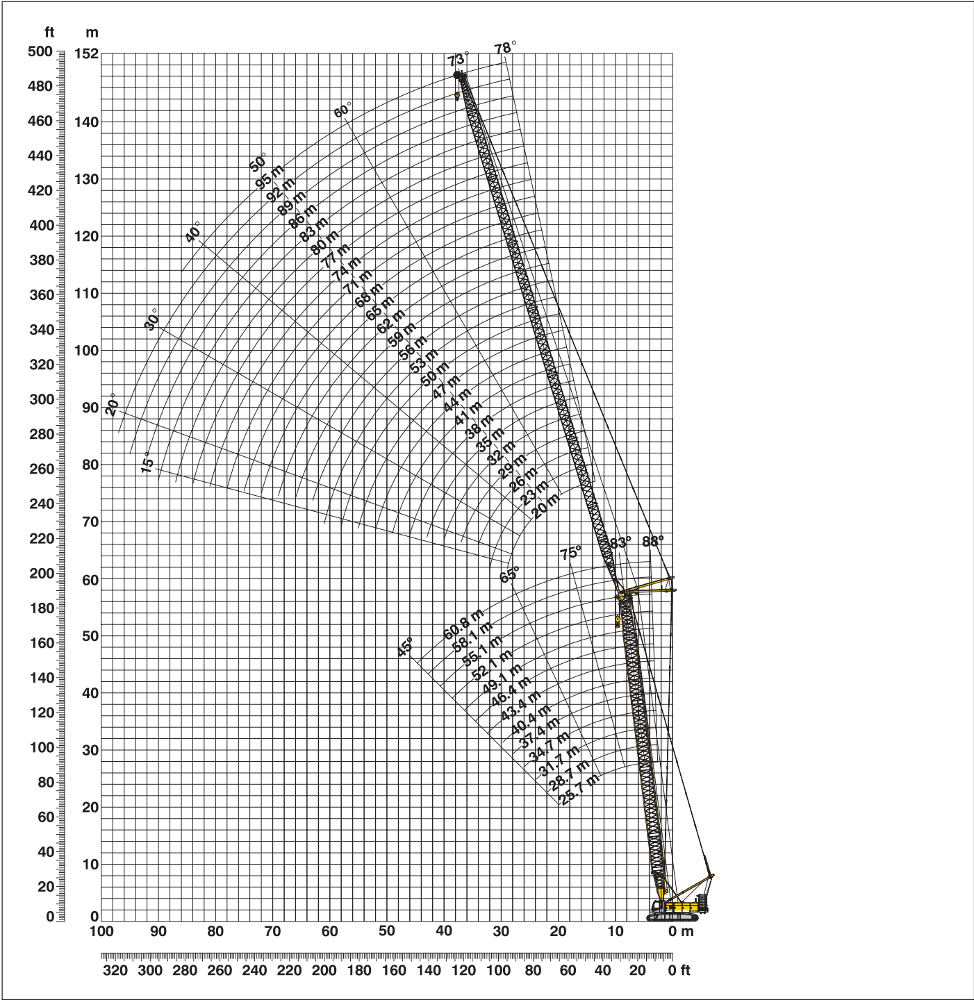
Auslegerzusammenbau für Hauptauslegerlängen von 25.7 m - 60.8 m – s. Tab. 1, Seite 10 Konfiguration mit verstellbarem Nadelausleger (20 m - 95 m)
