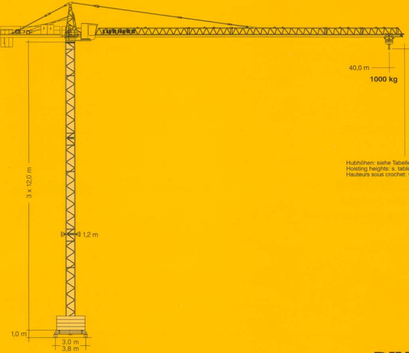
Turm 45 EC tower / le mât max. 36,1 m
