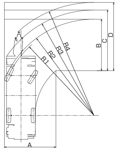
●前2輪ステアリング
