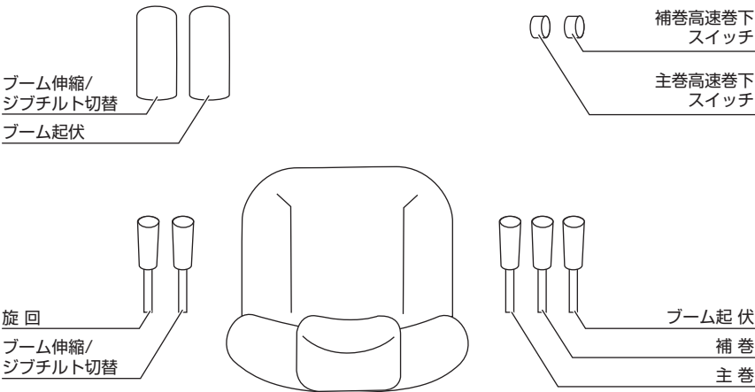
●標準仕様方式(ISO方式)
