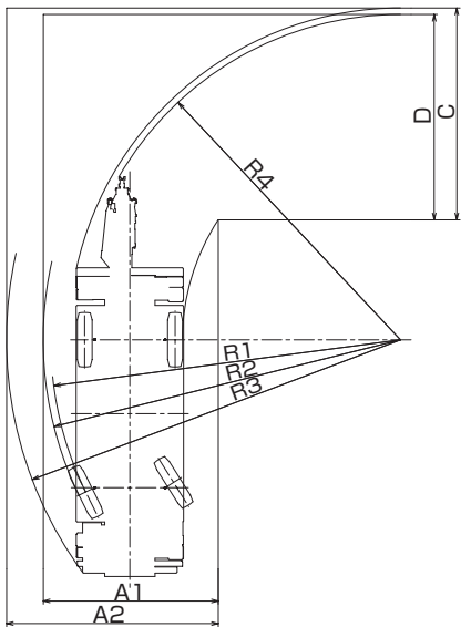
●後2輪ステアリング
