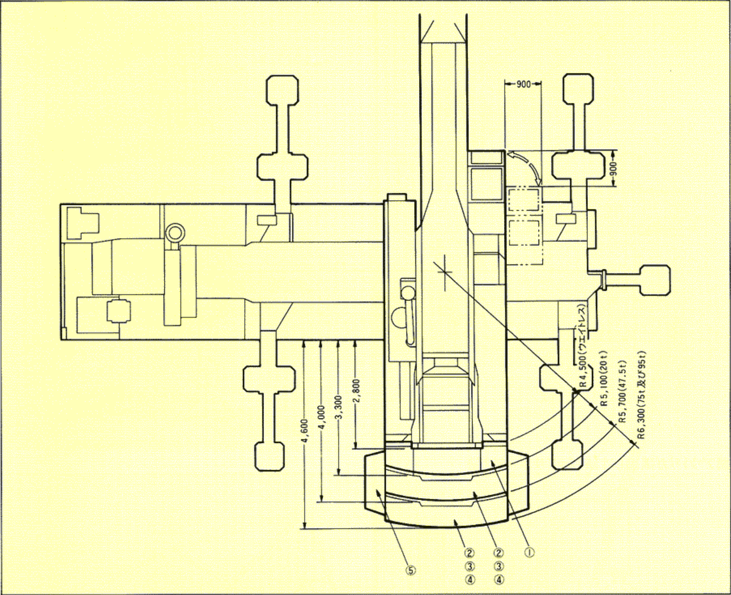
■外観寸法図
