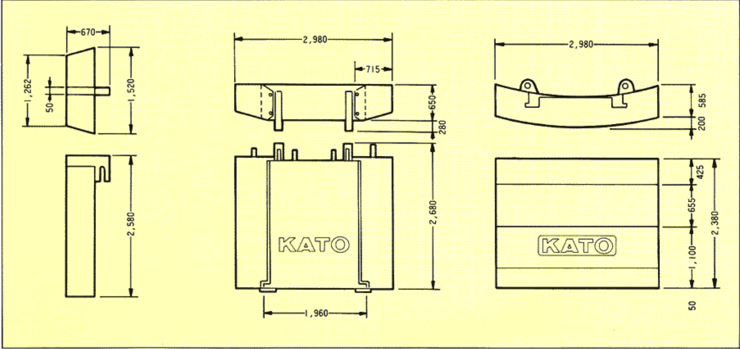
■外観寸法図
