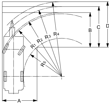
● 2輪ステアリングで右折する場合
