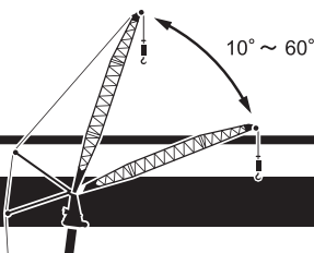
HA性能 40.9mブーム+4.4m+31.0mヘビーリフトジブ
