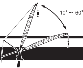
HA性能 40.9mブーム+4.4m+47.0mヘビーリフトジブ
