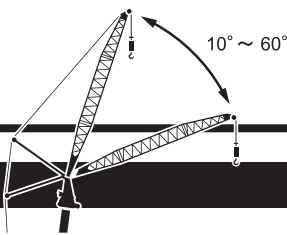
HA性能 40.9mブーム+4.4m+54.0mヘビーリフトジブ
