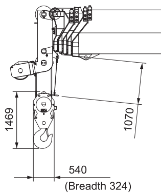
50 ton hook
