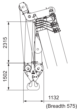
130 ton hook
