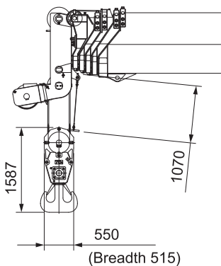
70 ton hook
