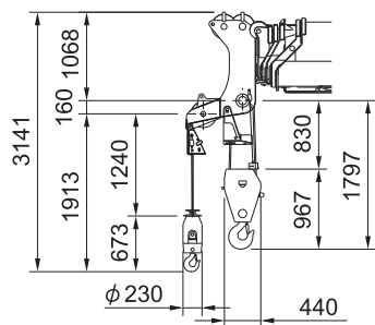
22ton hook
