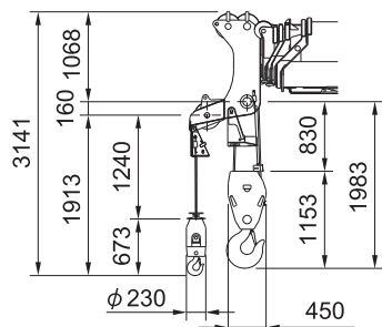
35ton hook
