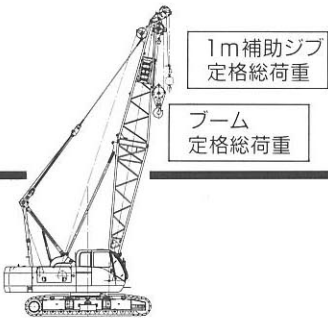
■ブーム定格総荷重表 (25.0ton カウンタウェイト装着時・全旋回) (単位: ton)
