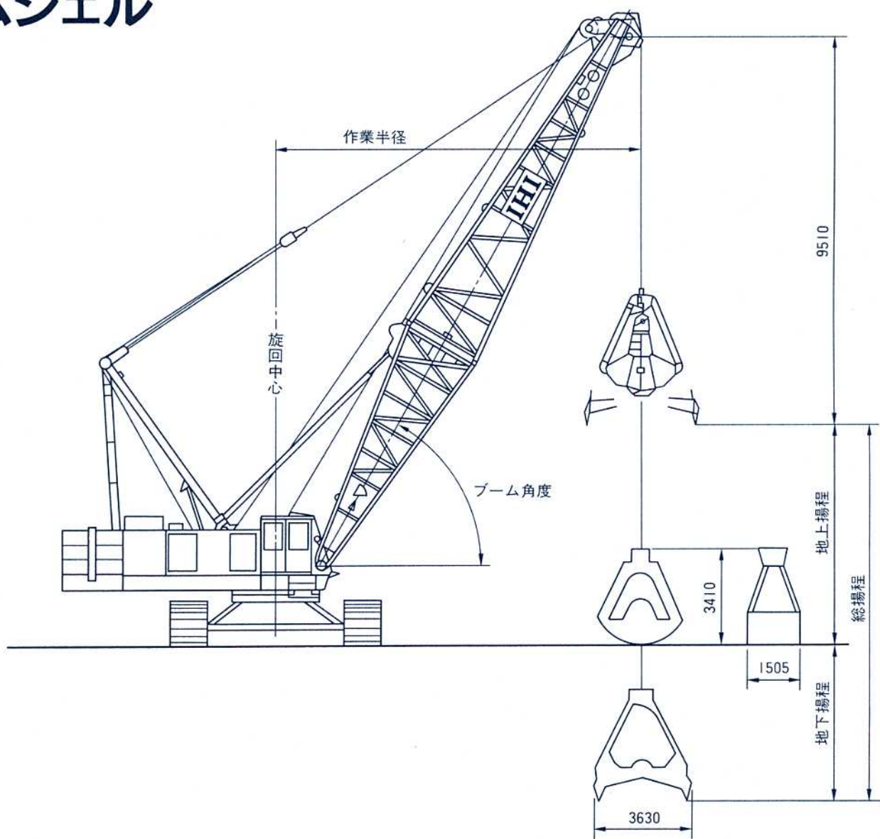
■外形寸法図 単位: mm
