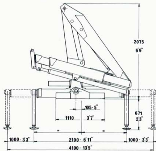
DIMENSIONS - afmetingen - DIMENSIONES
