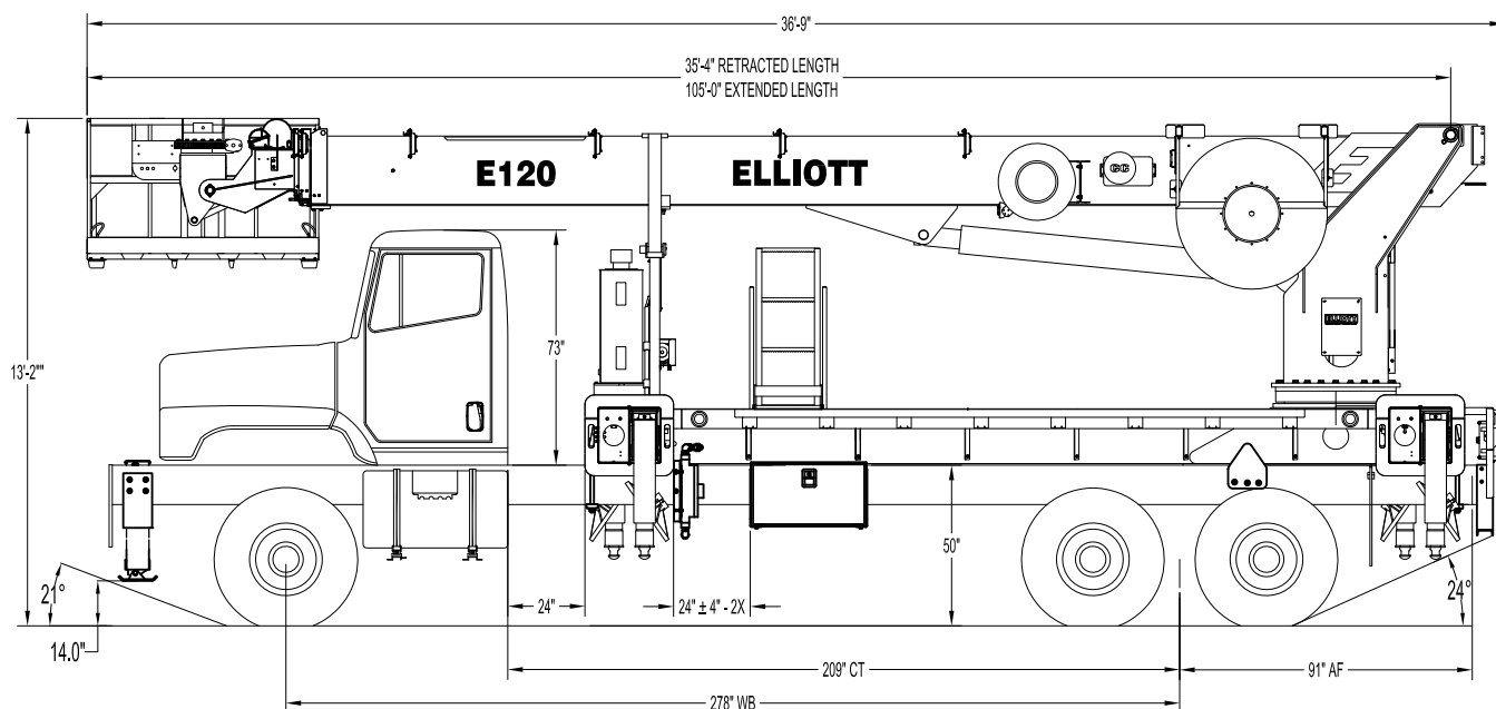
E120 SIDE VIEW DIAGRAM
