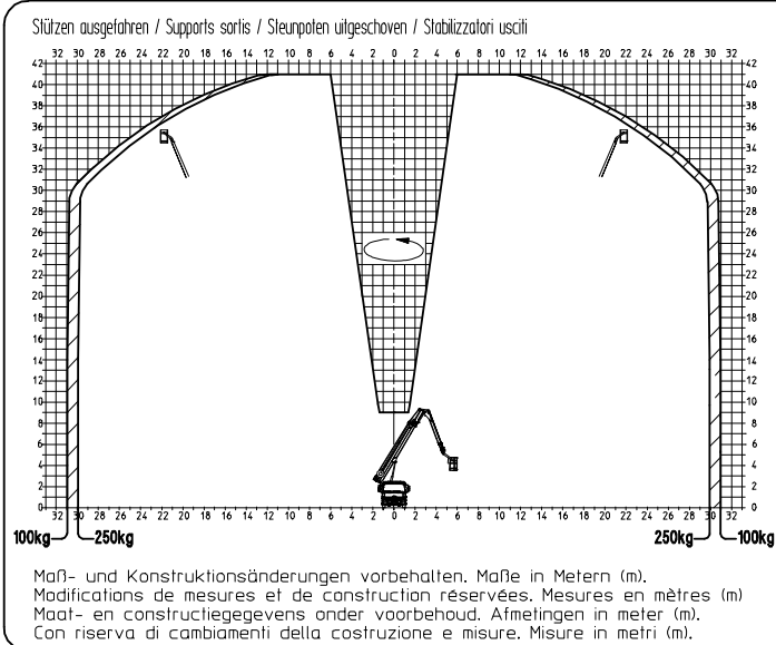
AK 41/6000 Max. Reichweiten bei ganz ausgefahrenen Stützen Maße in Meter (m). Maß- und Konstruktionsänderungen vorbehalten !
