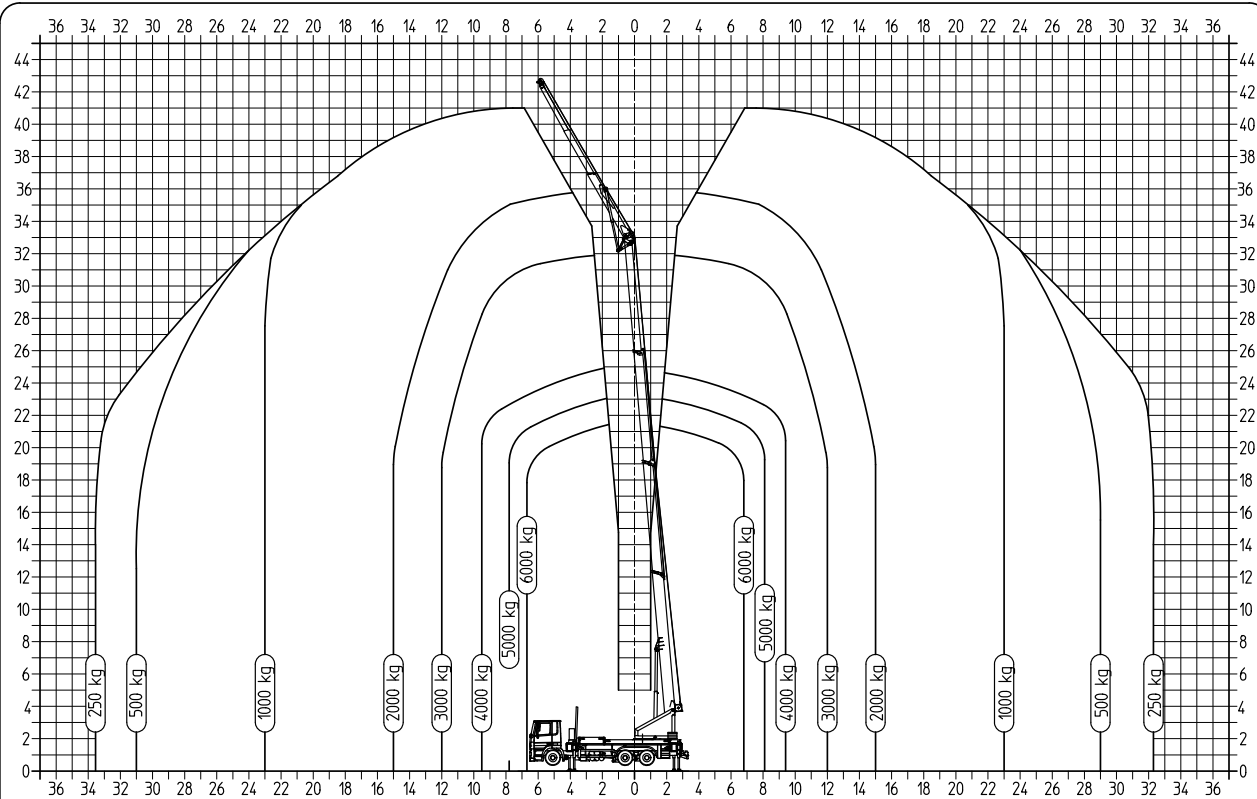
AK 41/6000 Max. Reichweiten bei ganz ausgefahrenen Stützen Maße in Meter (m). Maß- und Konstruktionsänderungen vorbehalten !
