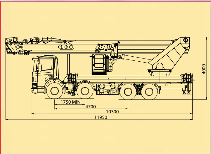
Ingombri su Strada - Road Overall Dimensions Dimensions Routieres - Abmessungen über alles
