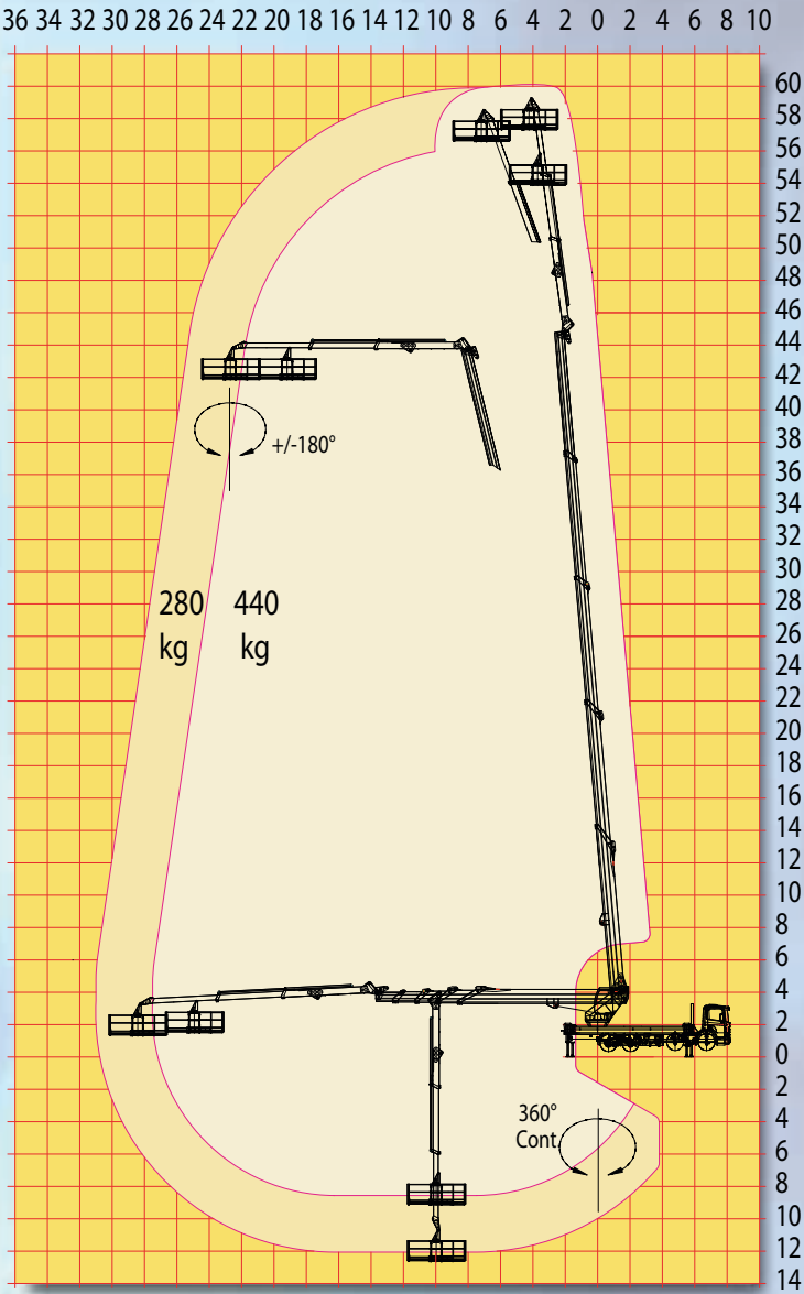
Campo di Lavoro - Work Range Diagram Champ de Travail - Arbeitsfeld
